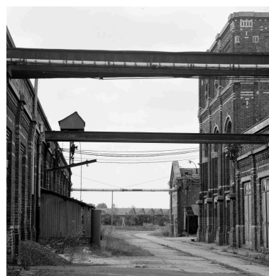
Vue vers le nord entre le tissage, à gauche, et la salle des machines, à droite, reliés par un palan monorail.
