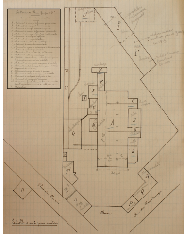
Plan général de l'usine en 1914, dressé en 1919 (AD Aisne). Phot. Pillet Frédéric IVR22_20060205364NUCAB
