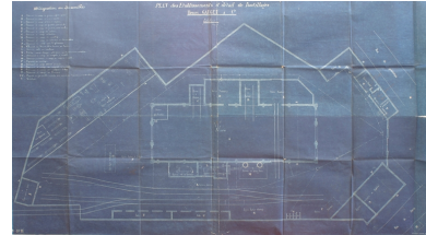
Plan général du site en 1919 (AD Aisne). Phot. Pillet Frédéric IVR22_20060205365NUCAB
