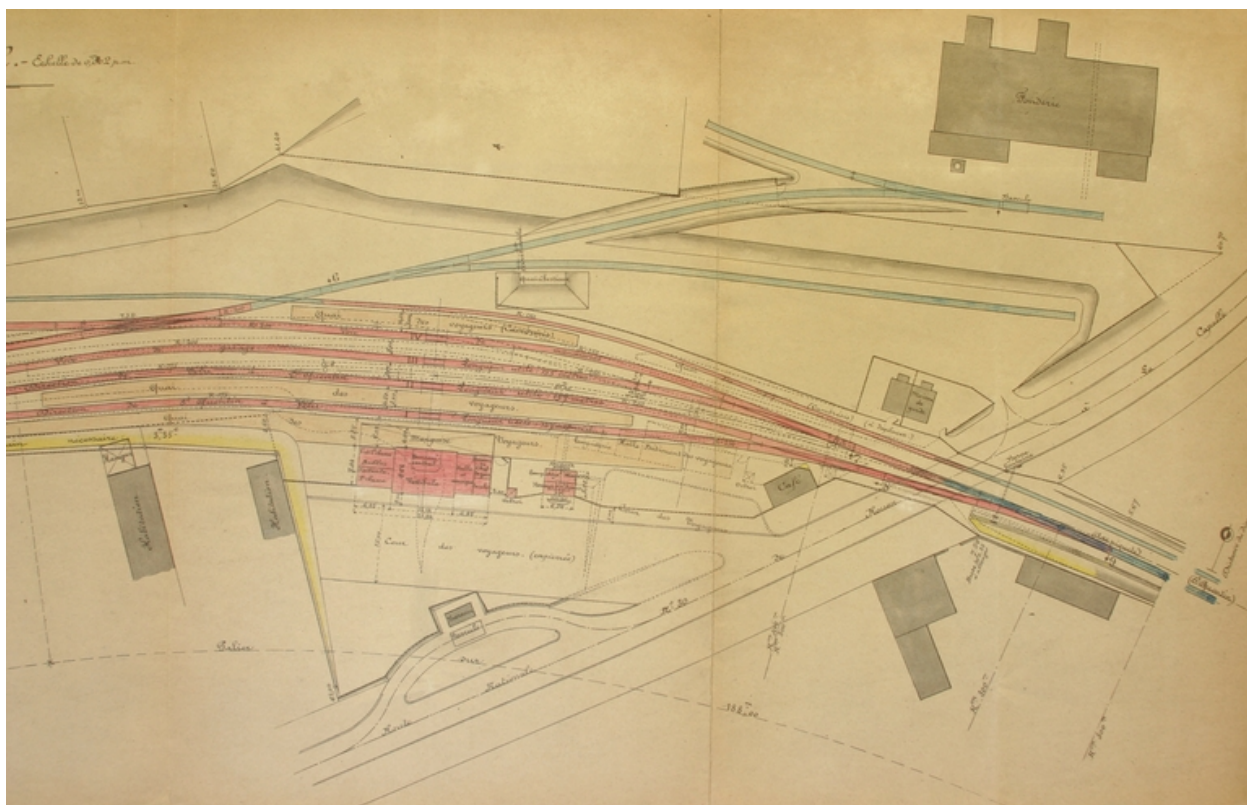
Plan masse de la gare de Rocourt (chemin de fer Vélizy-Bertincourt), de la fonderie et de son embranchement ferroviaire, 1913 (AC Saint-Quentin).
