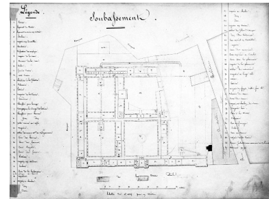
Plan de distribution générale du sous-sol, non daté (milieu du 19e siècle), avec légende indiquant l'affectation des différentes salles (AD du Nord. Fonds du CHR ; plan 2728).
