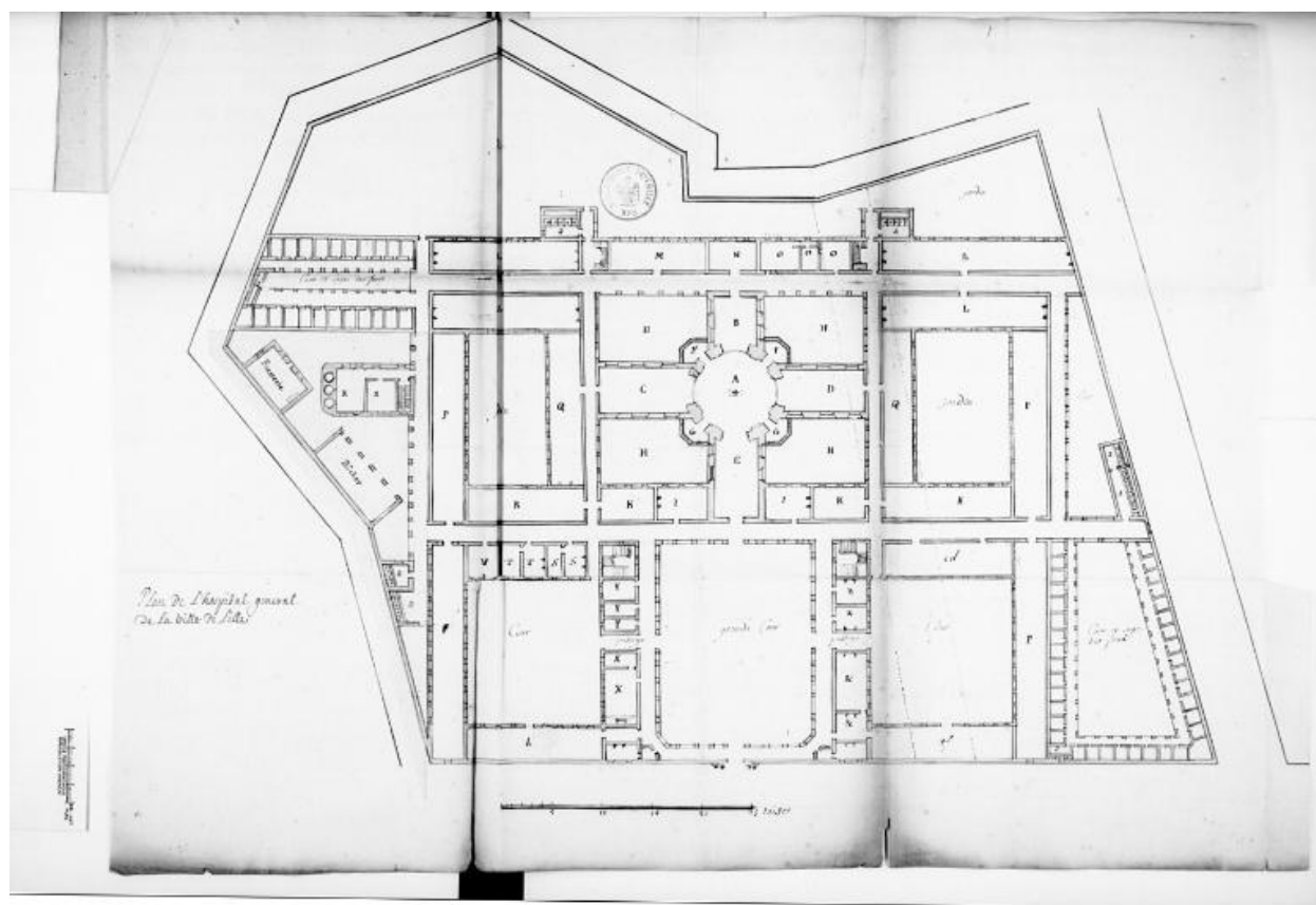
Plan de distribution générale du rez-de-chaussée correspondant vraisemblablement à un avant-projet, sans date, vers 1740.
