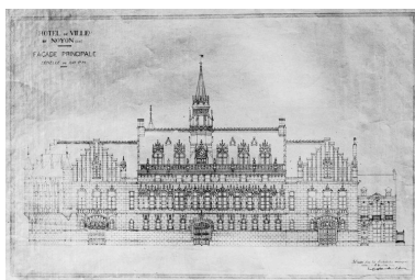
Projet de restauration. Elévation de la façade principale, par Chiffot et Lefèvre, 1922 (AC Noyon). Phot. Jean-Michel PERIN IVR22_19856000070XB
