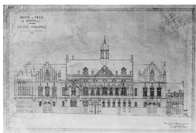
Projet de restauration. Elévation de la façade principale, par Chiffot et Lefèvre, 1928 (AC Noyon). Phot. Jean-Michel PERIN IVR22_19856000069XB
