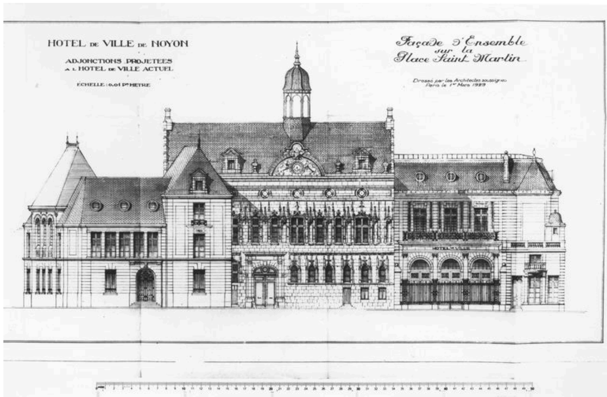
Elévation antérieure avec adjonctions projetées, par Chifflet et Lefèvre, 1929.
