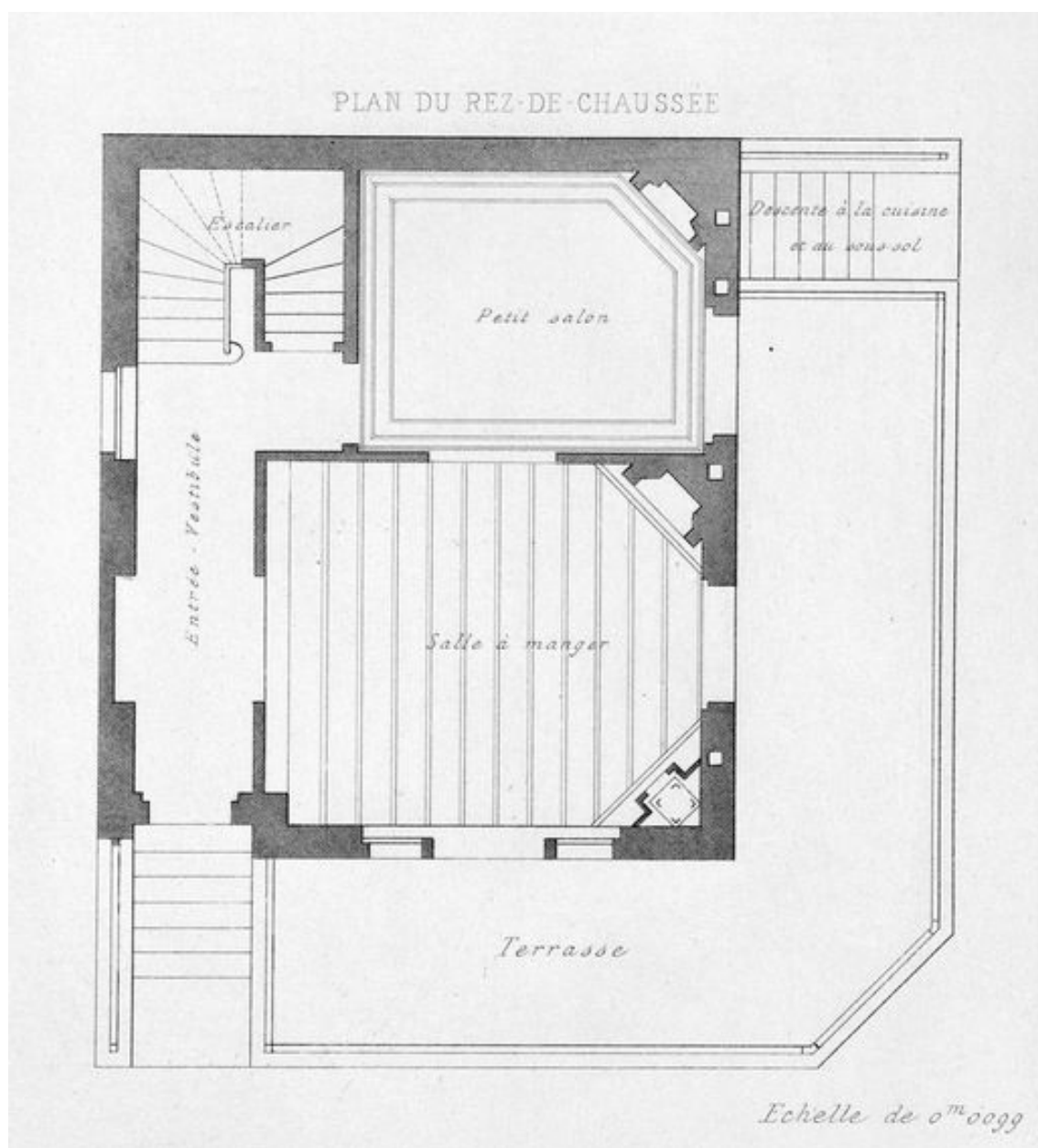
Villa Bambino, plan du rez-de-chaussée (AD Somme ; 1 J 3596/8).
