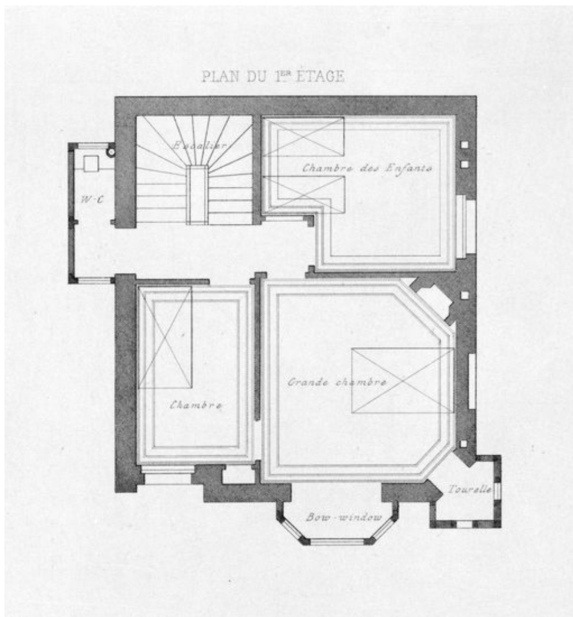
Villa Bambino, plan du premier étage (AD Somme ; 1 J 3596/8).
