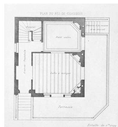
Villa Bambino, plan du rez-de-chaussée (AD Somme ; 1 J 3596/8).
