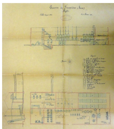
Plan de la sucrerie, 1902.
