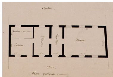
Plan du rez-de-chaussée, 1878 (AD Somme ; 99 T 3804 20/1). Phot. Archives départementales de la Somme IVR22_20038010167NUCA
