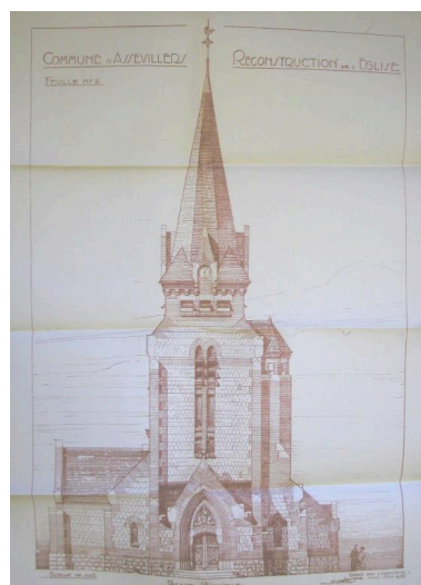
Projet de reconstruction de l'église : façade principale, feuille 2, Louis Duthoit, juin 1925 (AD Somme ; 10 R 140). Phot. Gilles-Henri Bailly (reproduction)
