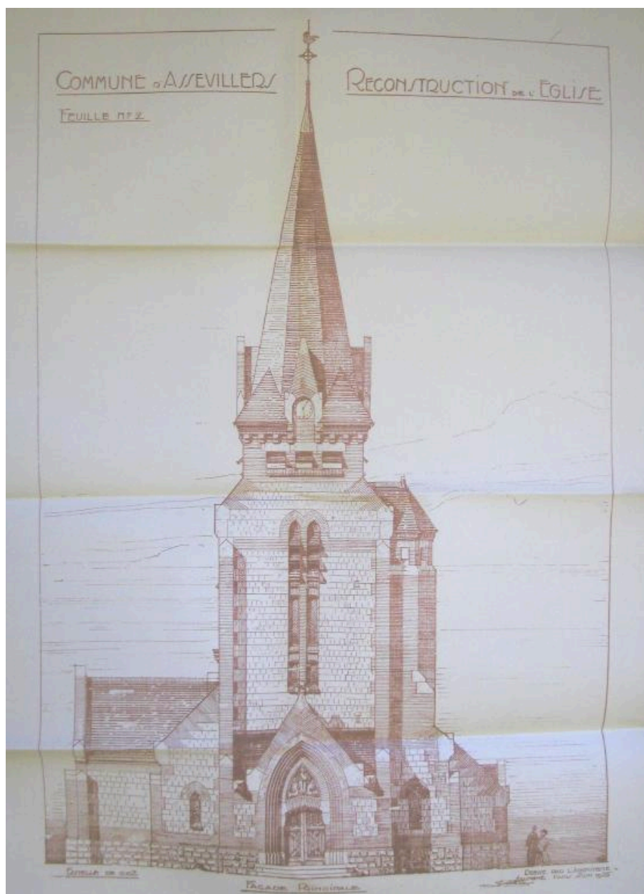
Projet de reconstruction de l'église : façade principale, feuille 2, Louis Duthoit, juin 1925 (AD Somme ; 10 R 140).
