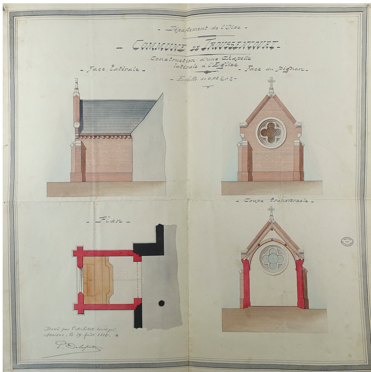
Église de Troussencourt (Oise). Plan, coupe, élévation pour la reconstruction de la chapelle, par Paul-Jules-Joseph Delefortrie, 1882
