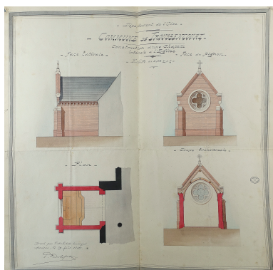
Église de Troussencourt (Oise). Plan, coupe, élévation pour la reconstruction de la chapelle, par Paul-Jules-Joseph Delefortrie, 1882 Repro. Marc Kérignard IVR32_20246000043NUCA
