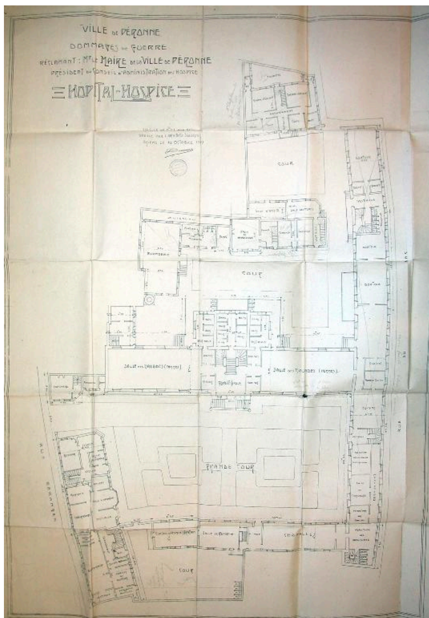
Hôpital-hospice de Péronne : plan d'ensemble du rez-de-chaussée, Darcourt (architecte), 10 octobre 1919 (AD Somme ; 10 R 1033).
