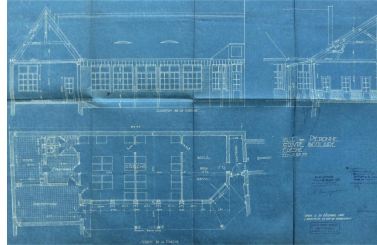
Ville de Péronne. Groupe scolaire. Crèche. Plan au sol, élévation et coupe, Jacques Debat-Ponsan architecte, 1925 (AD Somme ; 99O 3002). Phot. Isabelle Barbedor IVR32_20228005152NUCA
