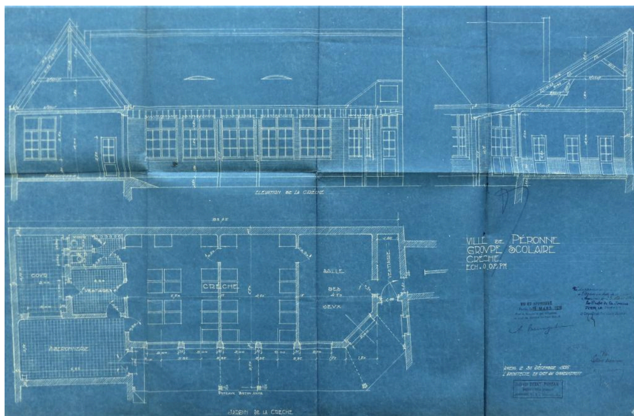
Ville de Péronne. Groupe scolaire. Crèche. Plan au sol, élévation et coupe, Jacques Debat-Ponsan architecte, 1925 (AD Somme ; 99O 3002).
