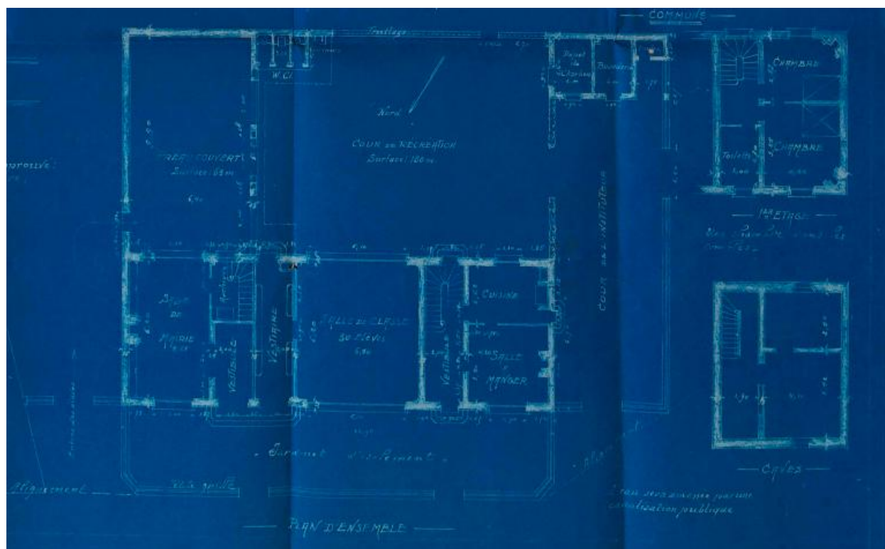
Poeuilly. Reconstruction des bâtiments communaux, plan d'exécution d'après C.-A. Dory, 1923 (AC Poeuilly). Vue de détail des plans.
