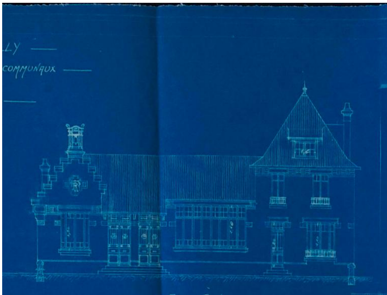
Poëuilly. Reconstruction des bâtiments communaux, plan d'exécution d'après C.-A. Dory, 1923 (AC Poëuilly). Vue de détail sur la façade.
