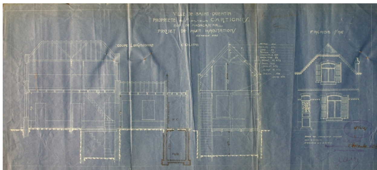
Façade antérieure et coupes, par Letrosne, 1921 (AC Saint-Quentin).
