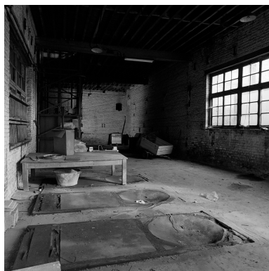
Atelier de crémage (A'). Au premier plan, le support des cuves. Phot. Olivier Marlard IVR31_19885902215X
