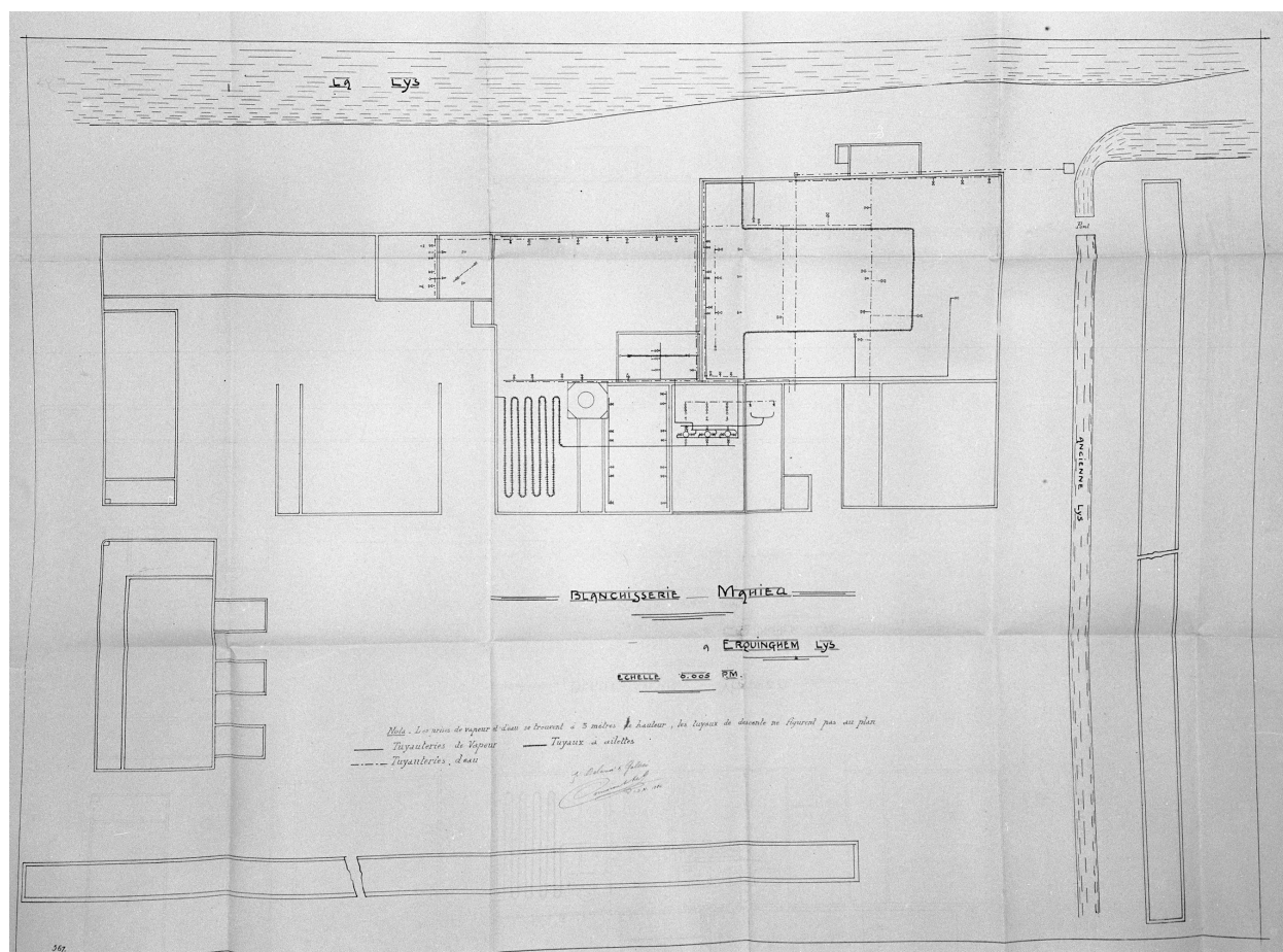
Plan de la tuyauterie, 1892 (AD Nord ; 10R5471).
