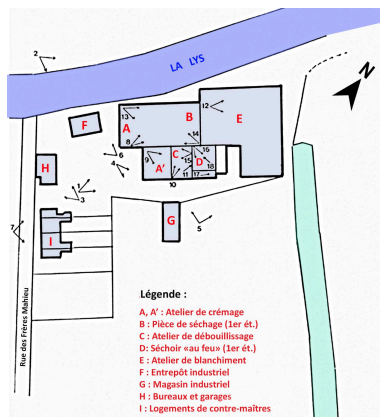
Plan masse avec angles de prise de vue d'après le plan cadastral de 1983, section B2. Dess. Jean-Marc Ramette IVR32_20235905030NUD
