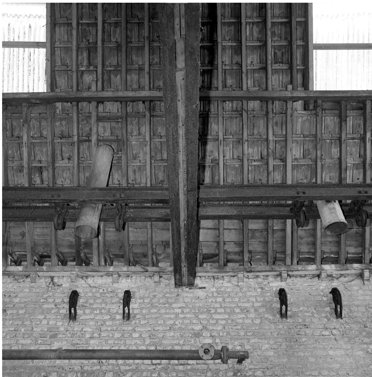
Atelier de débouillissage (C). Vestiges du mécanisme à contrepoids d'ouverture des cuves et cheminées d'évacuation.
