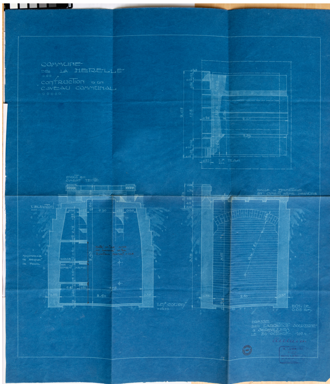
Coupes du projet de caveau communal par A. Lemaître, 1924 (AD Oise).
