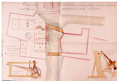
Plan de deux moulins à reviquer et à blé à construire dans l'île des Pestiférés, 1768 (AD Somme ; 1C CP 288/15).
