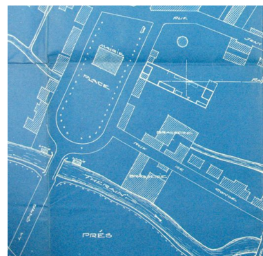
Plan de la brasserie : les bâtiments sont construits de part et d'autre du bras du bélier, 1923 (AD Oise ; 5MP2511).
