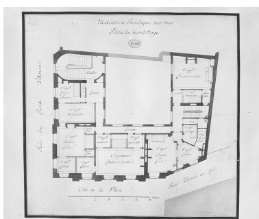
Plan du 2e étage. B.M. Boulogne- sur-Mer, 13e portefeuille, fol. 15. Phot. Jean-Michel Périn IVR31_19886200473X
