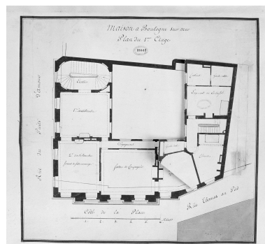
Plan du premier étage. B.M. Boulogne-sur-Mer, 13e portefeuille, fol. 14. Phot. Jean-Michel Périn IVR31_19886200488X
