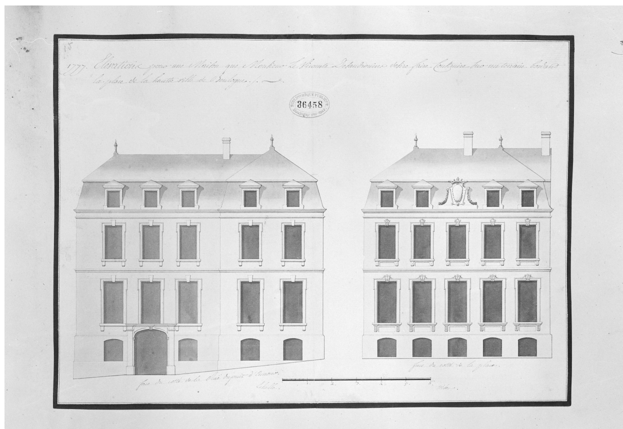
Premier projet (non exécuté), façades, dessin. B.M. Boulogne-sur-Mer, 13e portefeuille, fol. 15.
