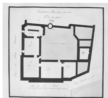
Plan du sous-sol. B.M. Boulogne- sur-Mer, 13e portefeuille, fol. 16. Phot. Jean-Michel Périn IVR31_19886200490X
