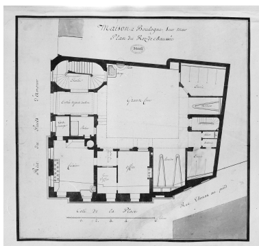
Plan du rez-de-chaussée. B.M. Boulogne-sur-Mer, 13e portefeuille, fol. 13. Phot. Jean-Michel Périn IVR31_19886200491X
