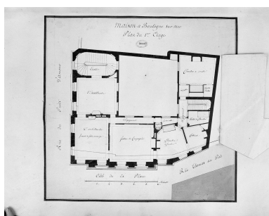
Plan du premier étage (variante). B.M. Boulogne-sur-Mer, 13e portefeuille, fol. 14. Phot. Jean-Michel Périn IVR31_19886200489X
