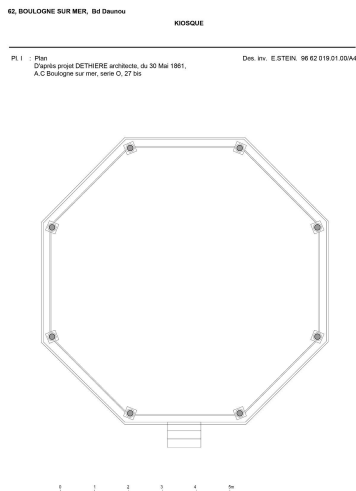
Plan du kiosque d'après le projet de l'architecte Dethière. Dess. Eddy Stein IVR32_19966200019NUD
