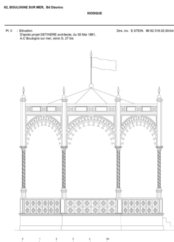
Dessin de l'élévation du kiosque d'après le projet de l'architecte Dethière. Dess. Eddy Stein IVR32_19966200018NUD
