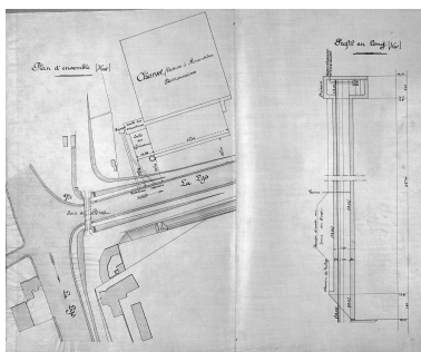
Charvet. Prise d'eau pour l'alimentation d'une machine à vapeur. Plan masse et de situation, coupe, 1897 (AD Nord ; S 3779). Repro. Philippe Dapvril
