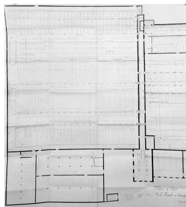
Charvet. Prise d'eau pour l'alimentation d'une machine à vapeur. Plan masse et de situation, coupe, 1897 (AD Nord ; S 3779). Repro. Philippe Dapvril
