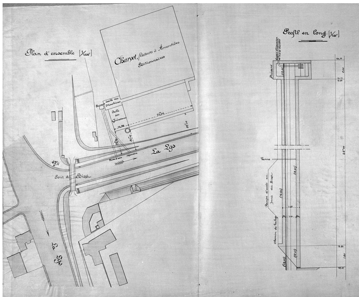
Charvet. Prise d'eau pour l'alimentation d'une machine à vapeur. Plan masse et de situation, coupe, 1897 (AD Nord ; S 3779).
