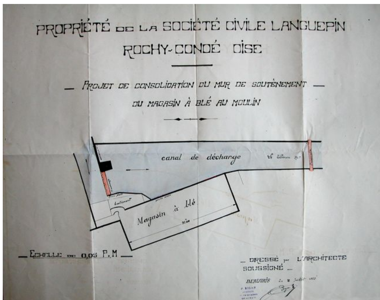
Plan partiel de la minoterie pour un projet de consolidation du mur du magasin à blé, par Paul Bigan, 1923.
