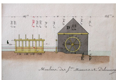
Profil du moulin à draps et à blé appartenant à Mineur et Delannoy, 1812.
