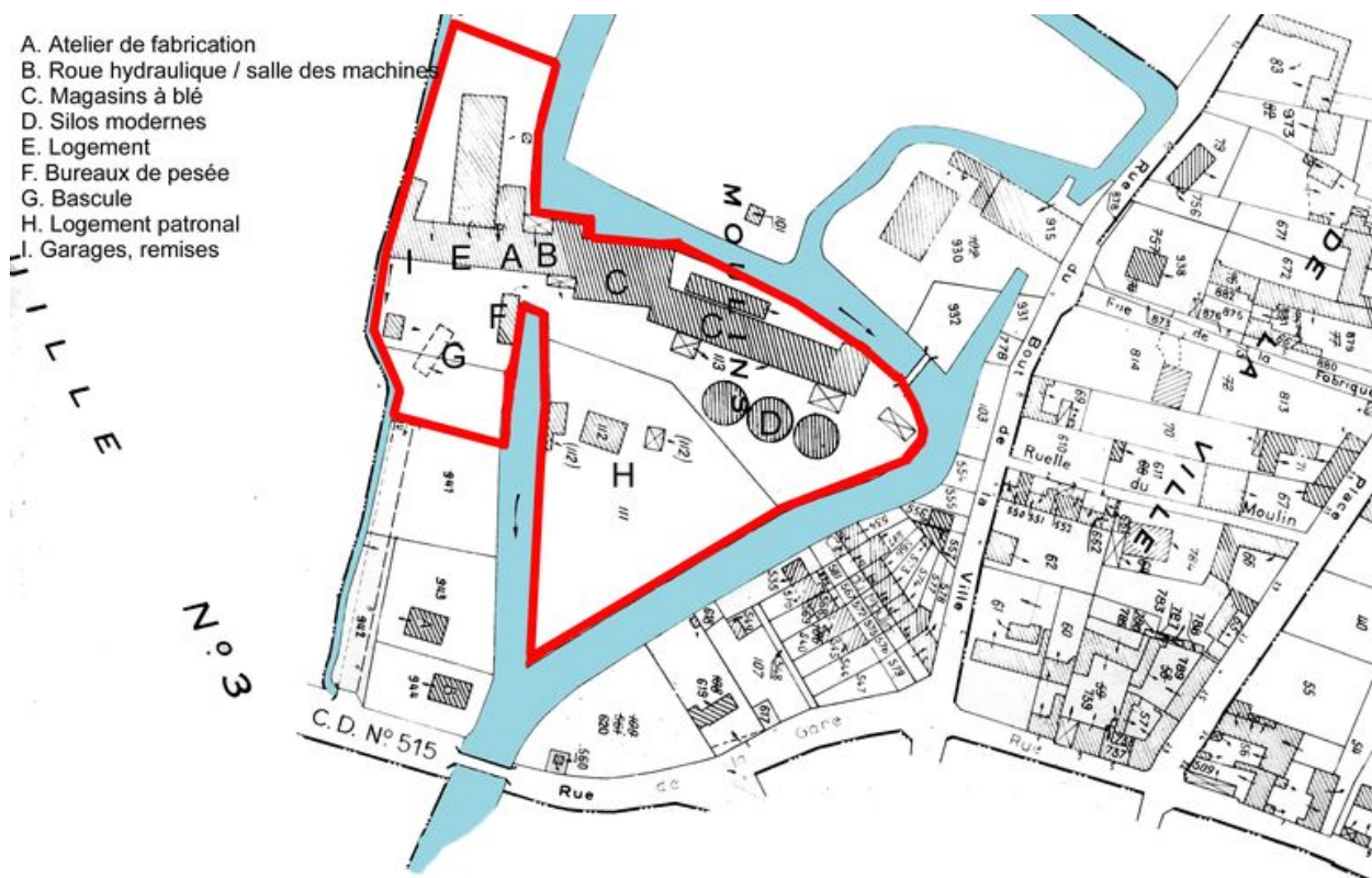
Plan masse de la minoterie avec indication de la fonction des bâtiments, extrait du plan cadastral communal.
