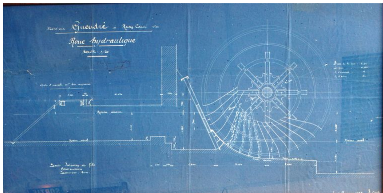
Coupe de la roue hydraulique.
