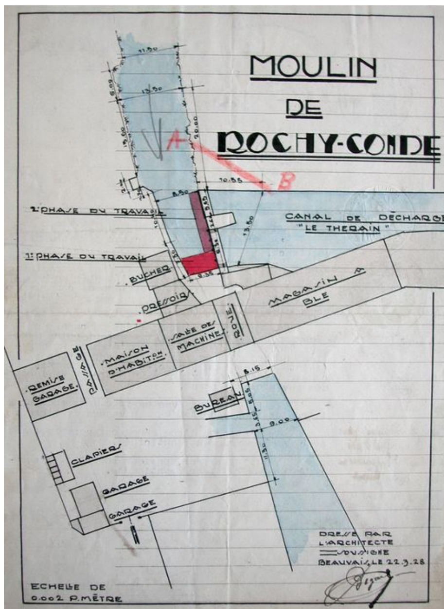
Plan détaillé du moulin de Rochy-Condé, par Paul Bigan, 1928.
