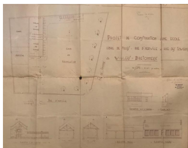
Projet de construction d'une école libre de filles. Plan d'ensemble, par Georges Bouffet architecte, 1930 (Archives paroissiales). Repro. Isabelle Barbedor IVR32_20208005265NUCA
