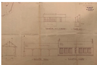
Projet de construction d'une école libre de filles. Elévations et coupes, par Georges Bouffet architecte, 1930 (Archives paroissiales). Repro. Isabelle Barbedor IVR32_20208005268NUCA
