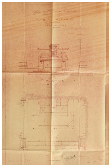
Église Saint-Nicolas de Bapaume - Autels latéraux (deux semblables) : élévation ; plan. Daté et signé Eugène Bidard (architecte), Soille (entrepreneur), 12 octobre 1933. (AD Pas-de-Calais, 20609/4). Phot. Thibaut Pierre (reproduction) IVR32_20216200081NUCA
