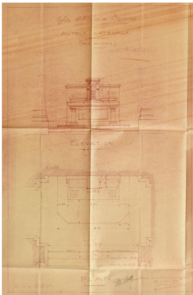
Église Saint-Nicolas de Bapaume - Autels latéraux (deux semblables) : élévation ; plan. Daté et signé Eugène Bidard (architecte), Soille (entrepreneur), 12 octobre 1933. (AD Pas-de-Calais, 2O609/4).
