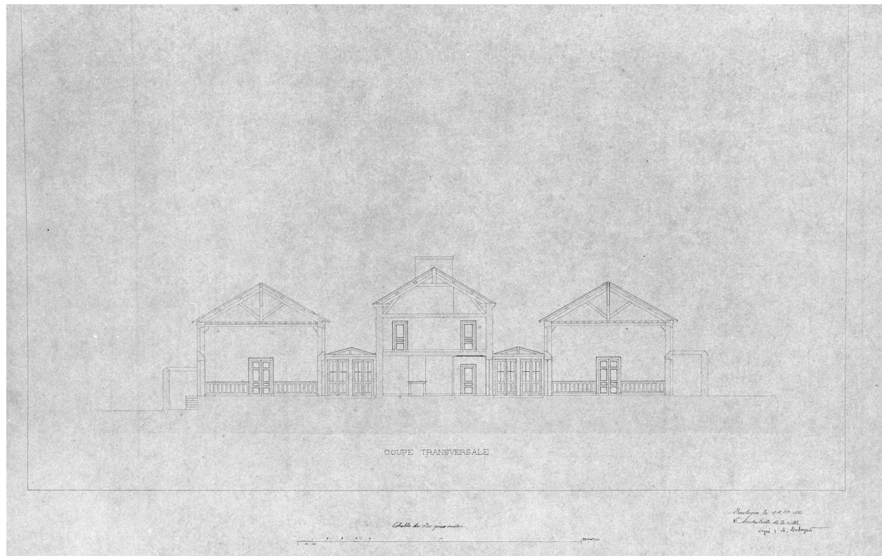
Coupe transversale. B.M. Boulogne-sur-Mer, mss. 535 P, pl. 34.
