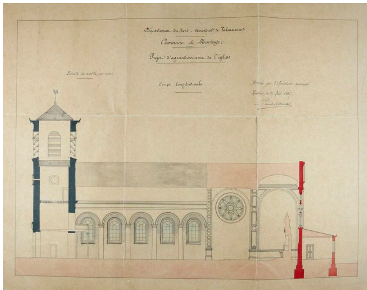
Coupe transversale, Paul Destombes architecte, 1888 (AD Nord 2O421-83).
