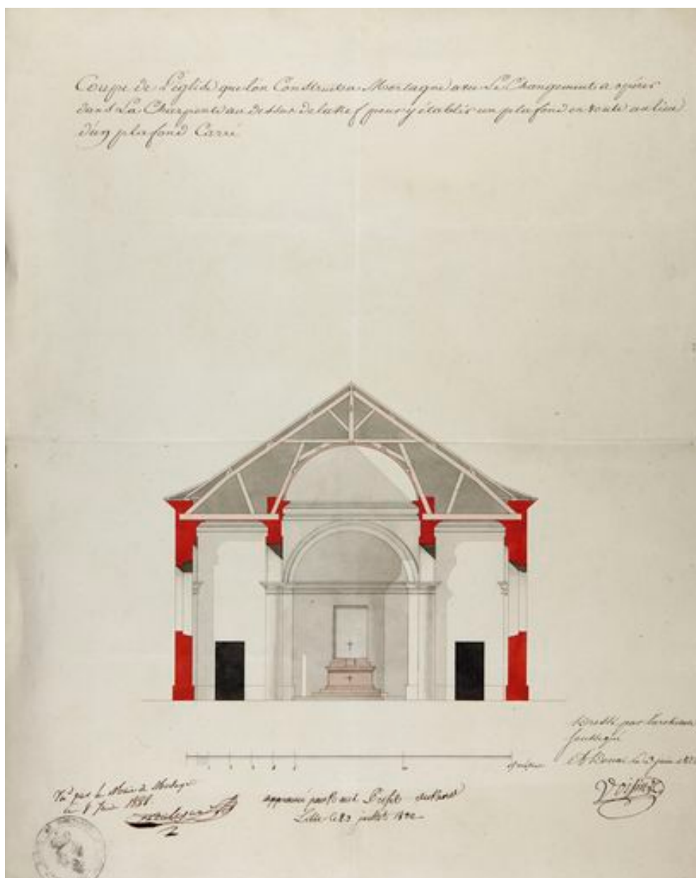
Coupe de l'église projetée, Voisin architecte (AD Nord 2O421-72).
