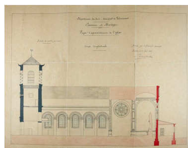
Coupe transversale, Paul Destombes architecte, 1888 (AD Nord 20421-83).
