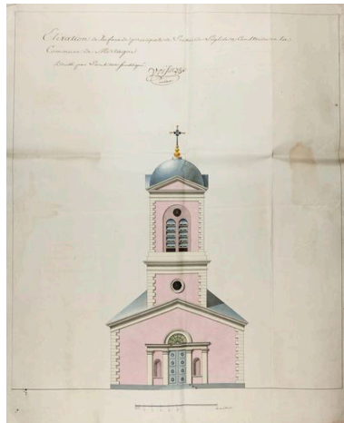
Elévation antérieure de l'église projetée, Voisin architecte, 1820 (AD Nord, 2O421-72). Phot. Hubert Bouvet IVR31_20105900557NUCA
