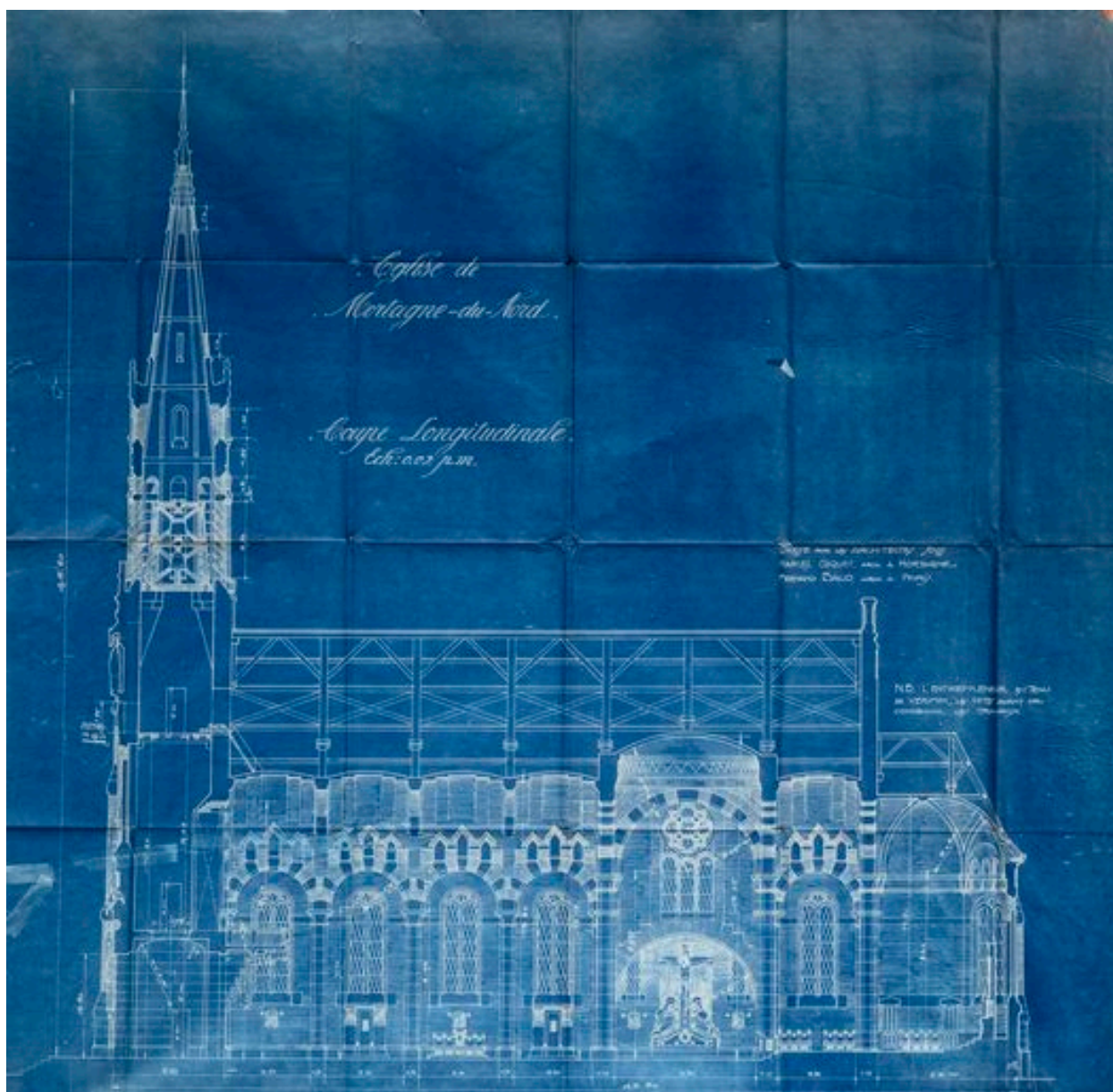
Coupe de l'église, Fernand Baud et Marcel Coquet architectes, 1924 (AD Nord, 2O421/200).
