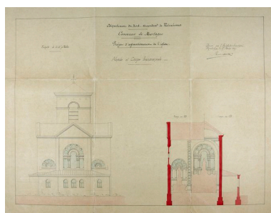
Elévation postérieure, Paul Destombes architecte, 1888 (AD Nord 20421-83).
