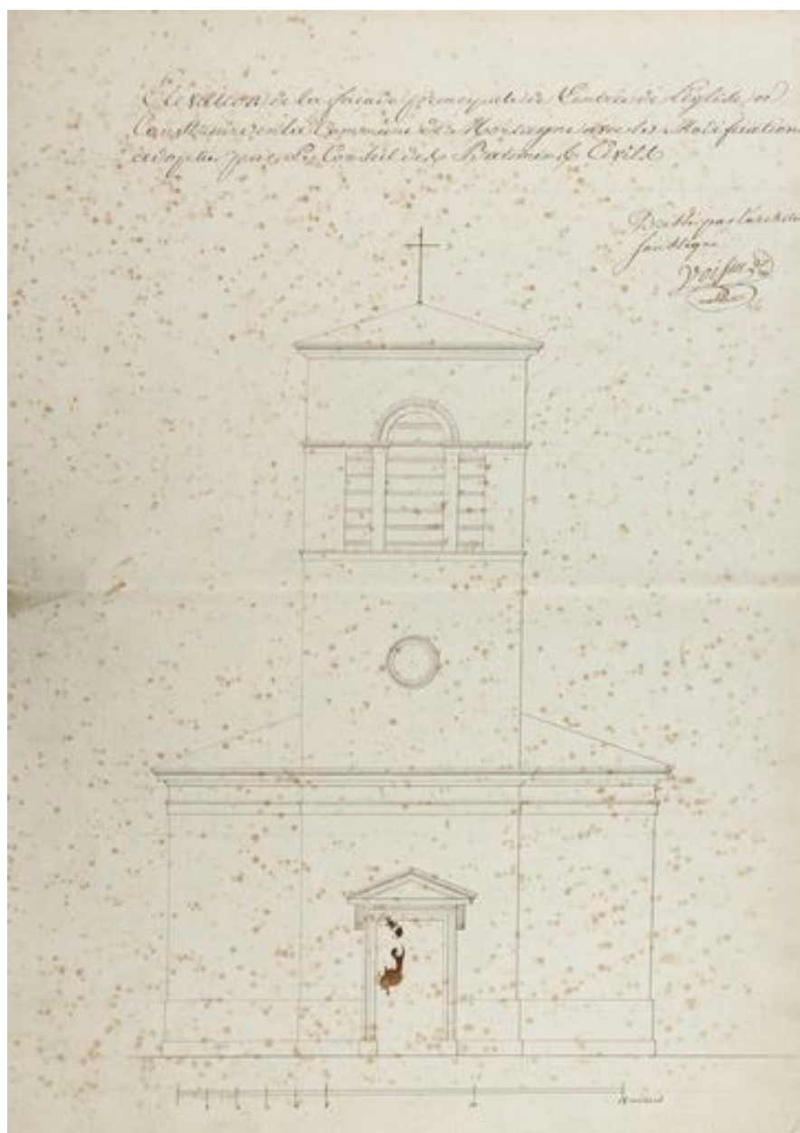
Elévation antérieure adoptée après modification, Voisin architecte (AD Nord, 2O421-75)
