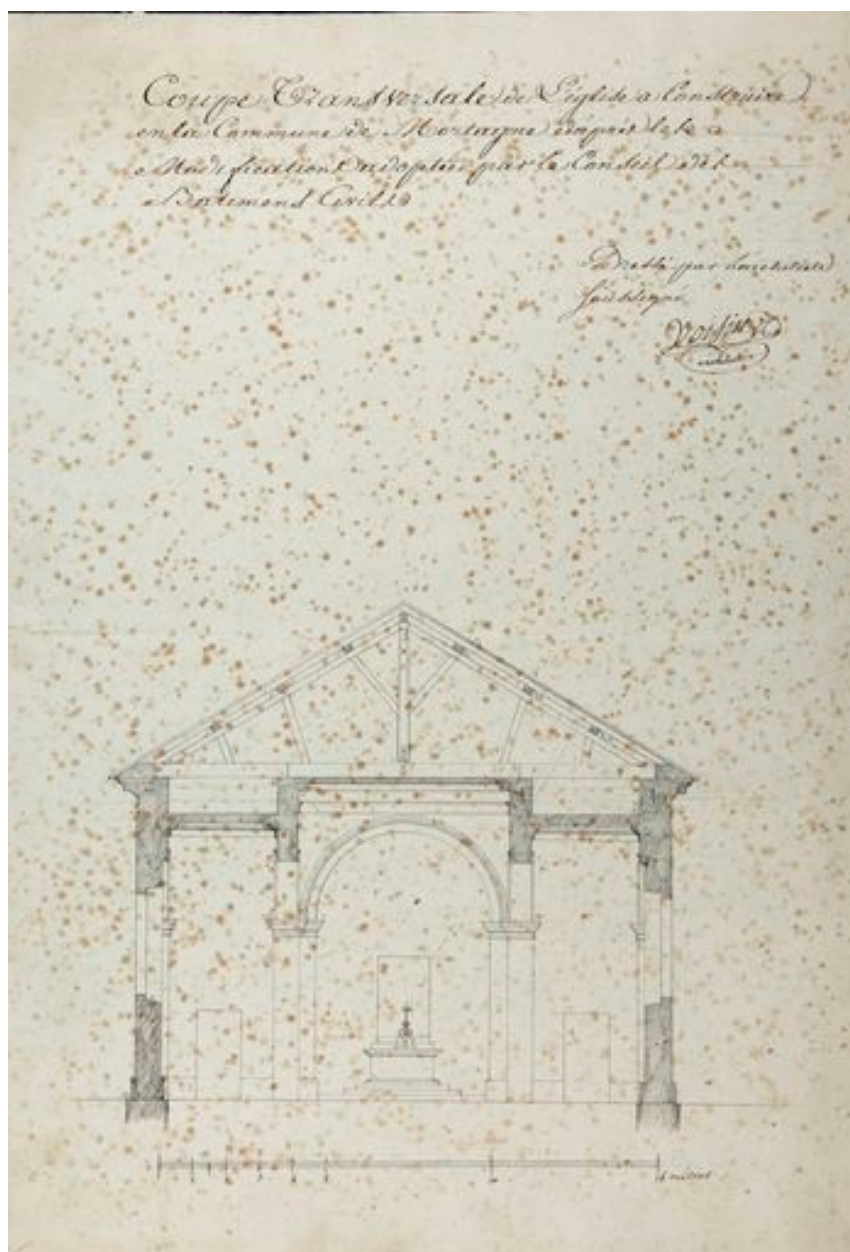
Coupe du parti adopté, Voisin architecte (AD Nord 2O421-75).
