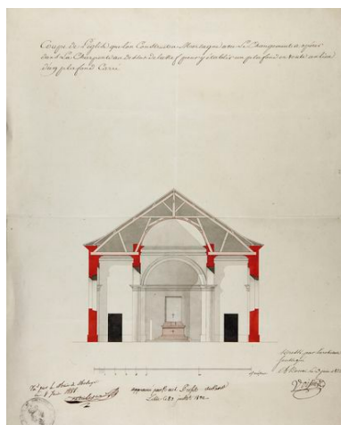
Coupe de l'église projetée, Voisin architecte (AD Nord 20421-72).
