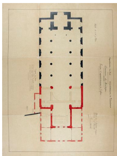
Plan du projet d'agrandissement, Paul Destombes architecte, 1888 (AD Nord 20421-83).
