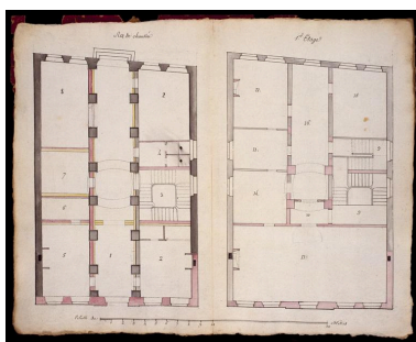
Plans du rez-de-chaussée et du 1er étage de l'hôtel de ville de Vervins : projet de réhabilitation non suivi d'exécution, vers 1820. Phot. Thierry Lefébure IVR22_19990207197XA
