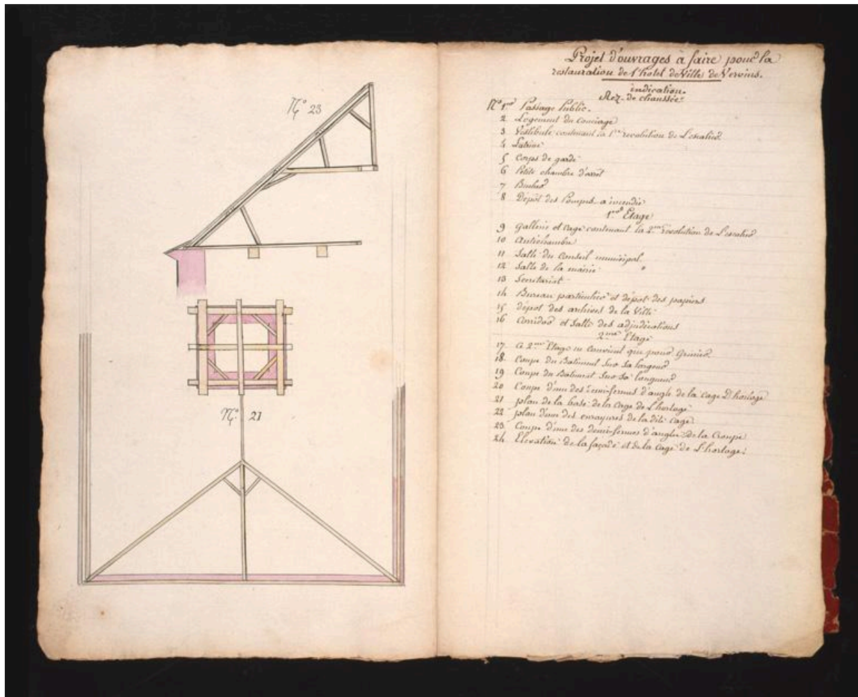
Plan de la base de la tour de l'horloge et coupe d'une demi-ferme de l'hôtel de ville de Vervins : projet de réhabilitation non suivi d'exécution, vers 1820.
