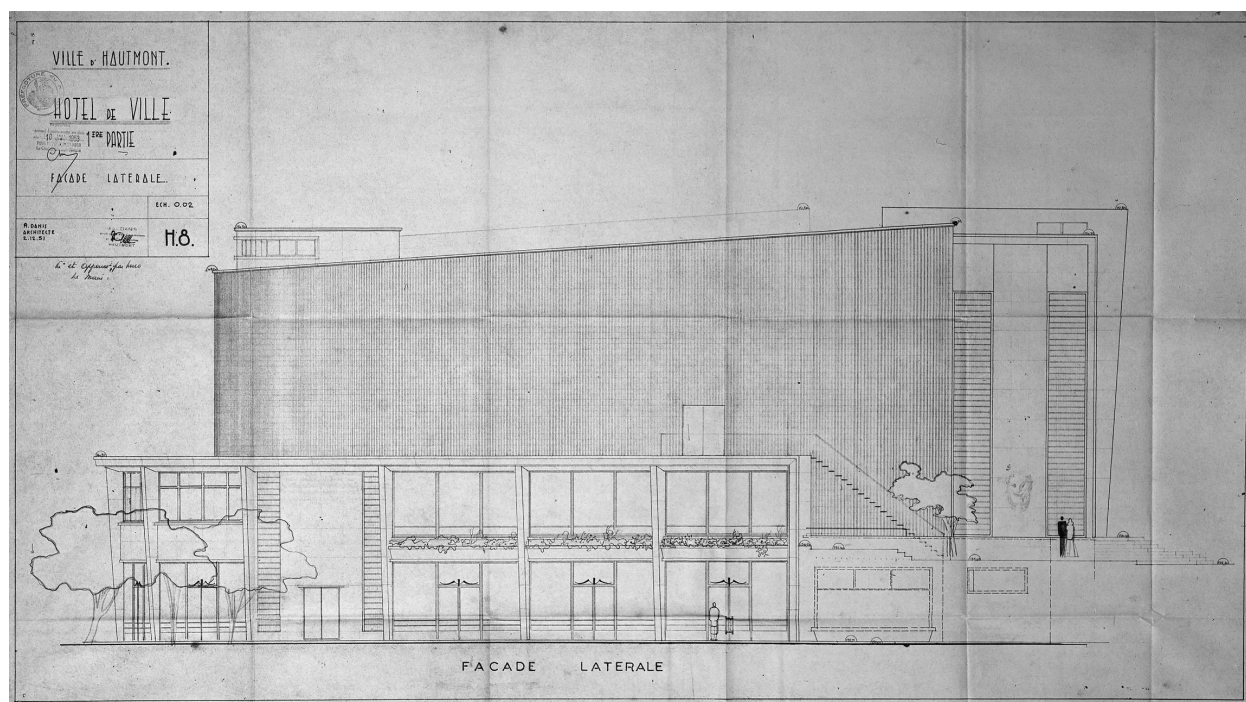
Élévation latérale de la salle des fêtes par Adolphe Danis (1886-1969), architecte, 1951 (AC Hautmont ; dossier centre culturel).
