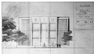
Élévation antérieure de la salle des fêtes par Adolphe Danis (1886-1969), architecte, 1951 (AC Hautmont ; dossier centre culturel). Repro. Olivier Marlard IVR31_19935900198V
