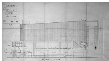
Élévation latérale de la salle des fêtes par Adolphe Danis (1886-1969), architecte, 1951 (AC Hautmont ; dossier centre culturel). Repro. Olivier Marlard IVR31_19935900196V
