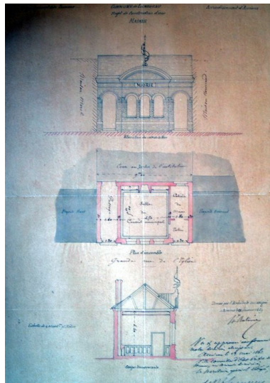
Longueau. Projet de construction d'une mairie, Henry Antoine architecte, 1859 (AD Somme ; 99 O 2405). Repro. Isabelle Barbedor IVR22_20058010503NUCA
