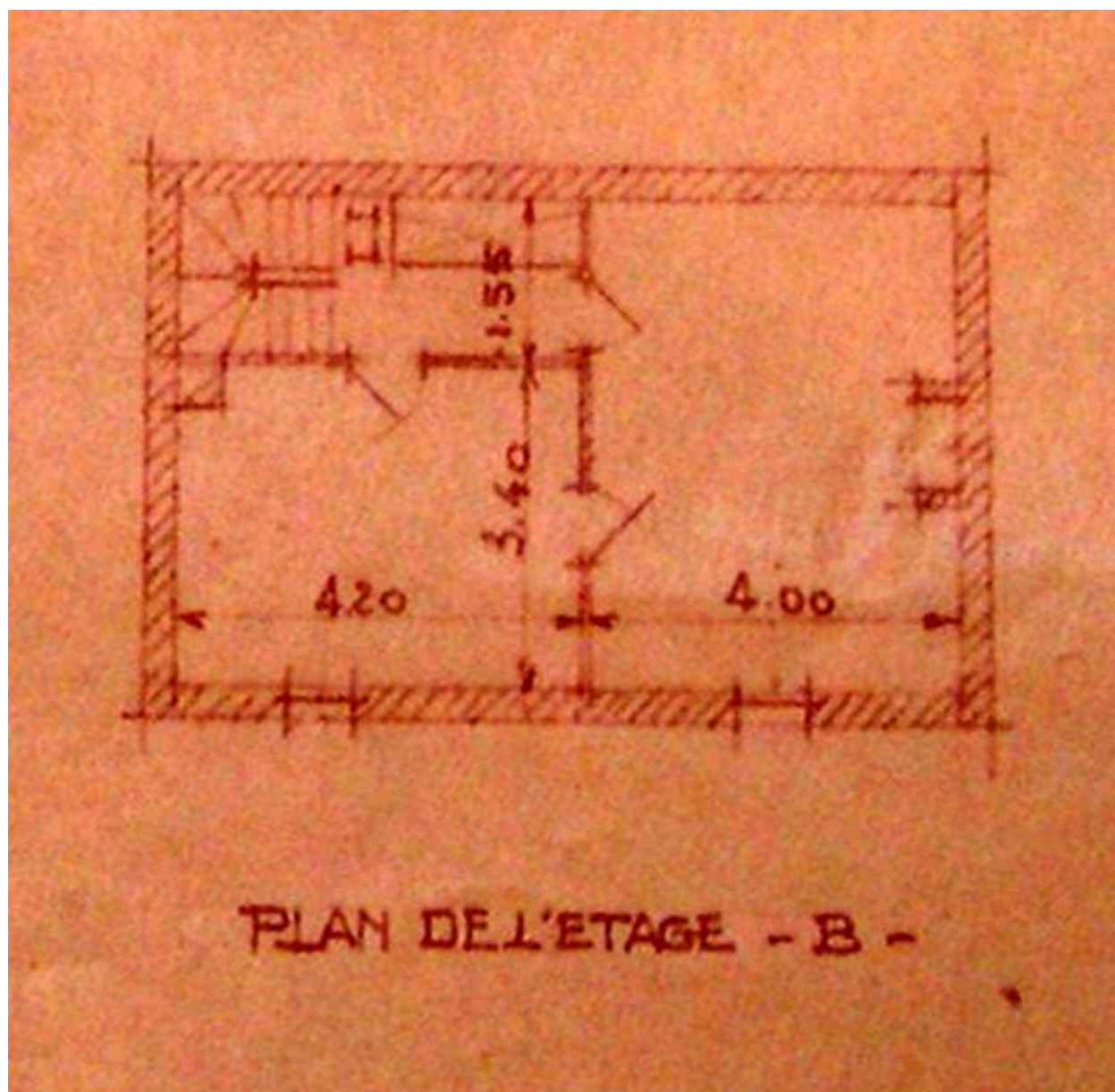
Logement. Plan de l'étage, 1934 (AD Somme ; 99 O 2406).
