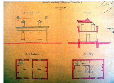
Longueau. Construction d'une maison d'habitation pour l'instituteur, Henry Antoine architecte, 1859 (AD Somme ; 99 O 2405). Repro. Isabelle Barbedor IVR22_20058010504NUCA
