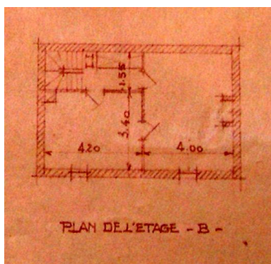
Logement. Plan de l'étage, 1934 (AD Somme ; 99 O 2406). Repro. Isabelle Barbedor IVR22_20048010488NUCA
