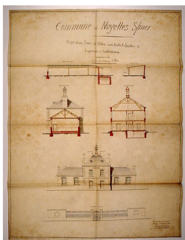
Projet d'une classe enfantine en 1882, par Alfred Marchand. Phot. Irwin Leullier IVR22_20068000069XAB
