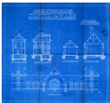
Coupe et élévation de l'école de filles. Phot. Monnehay-Vulliet Marie-Laure IVR22_20068000010XAB
