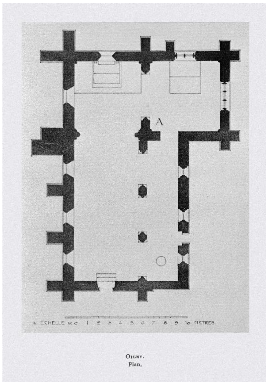
Plan de l'église, relevé par Étienne Moreau-Nélaton vers 1914 (Les Églises de chez nous. Arrondissement de Soissons, t. 2).
