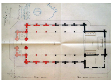
Plan d'achèvement de l'église, 1886 (AD Somme : 5V 612). Phot. Isabelle Barbedor IVR22_20068010052NUCA
