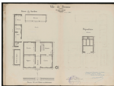
Ville de Péronne. Cimetière. Maison du gardien et dépositoire. Plan au sol. Coulombel conducteur des travaux, 1920 (AD Somme ; 10R 1008). Phot. Archives départementales de la Somme IVR32_20228005042NUCA
