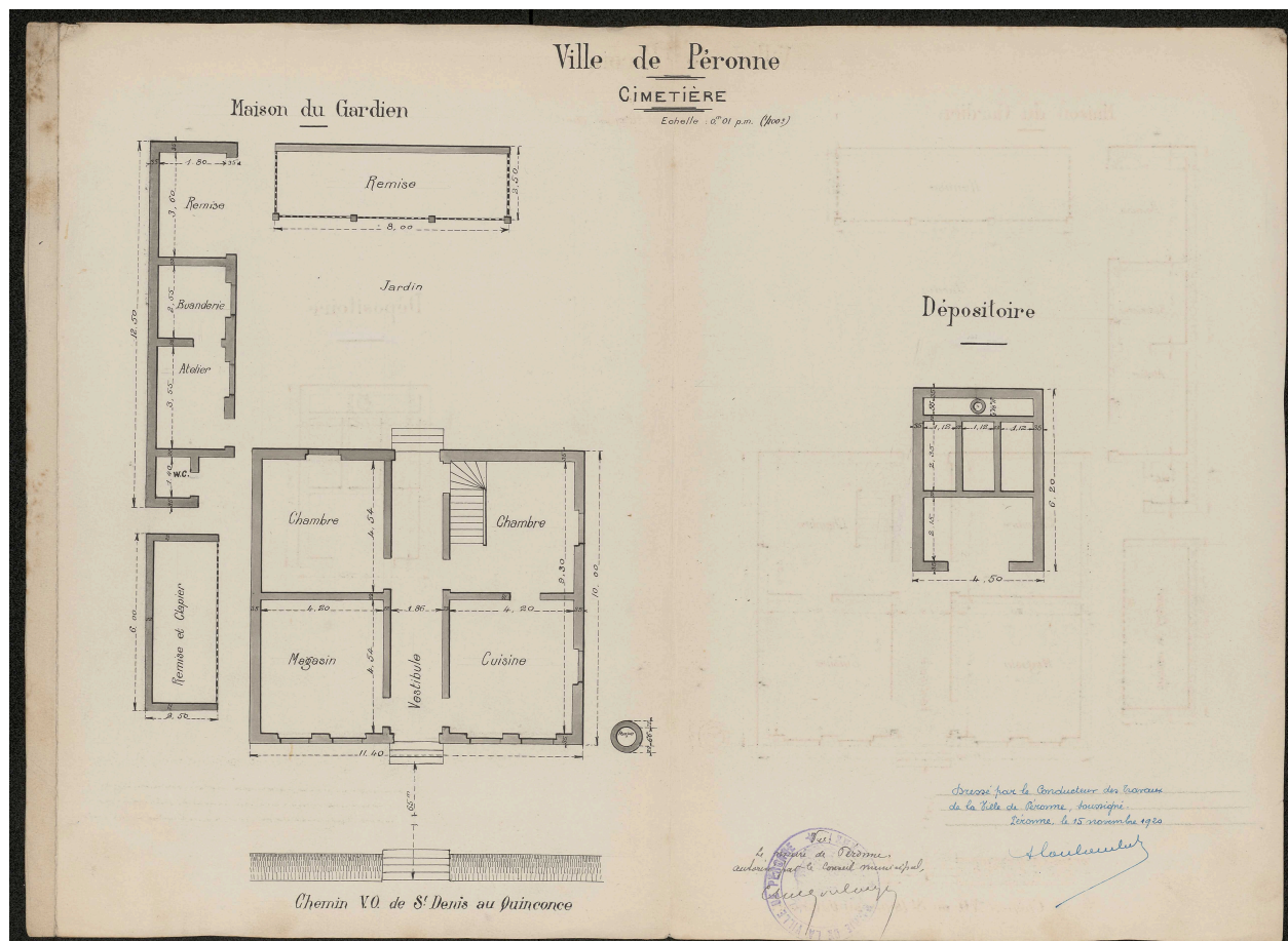
Ville de Péronne. Cimetière. Maison du gardien et dépôt. Plan au sol. Coulombel conducteur des travaux, 1920 (AD Somme ; 10R 1008).
