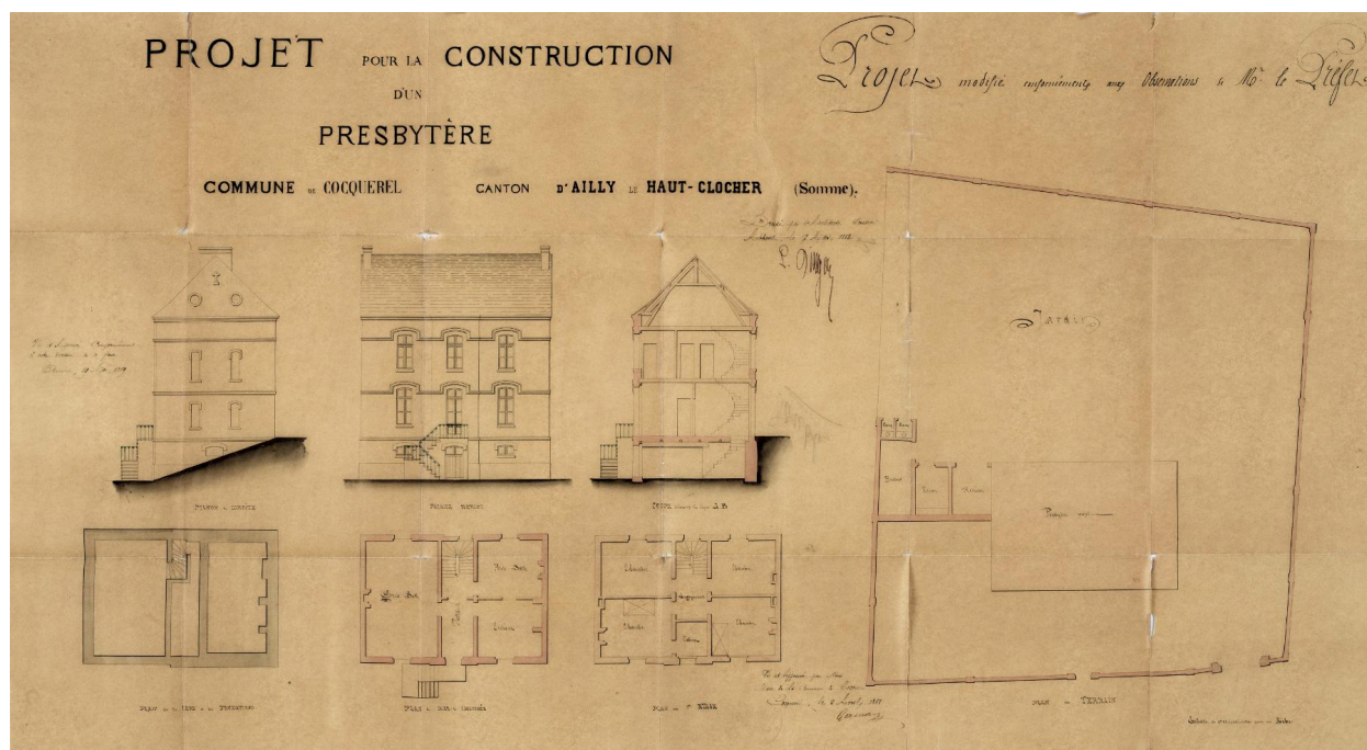
Projet pour la construction d'un presbytère, commune de Cocquerel. Léopold Digeon, architecte à Abbeville, mai 1868 (AD Somme ; 99 O 1185).
