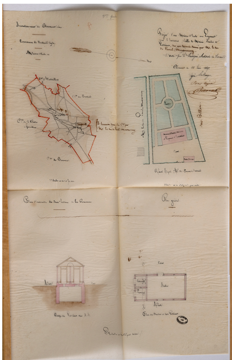
Vendeuil-Caply (Oise). Projet de mairie-école, plan de situation et plan du bucher, 1847 (AD Oise).
