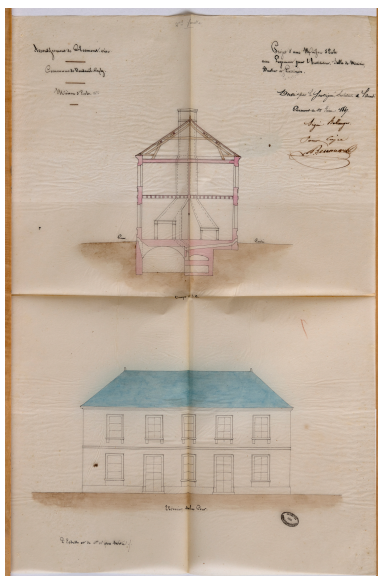
Vendeuil-Caply (Oise). Projet de mairie-école, 1847 (AD Oise). Repro. Marc Kérignard IVR32_20246001231NUCA
