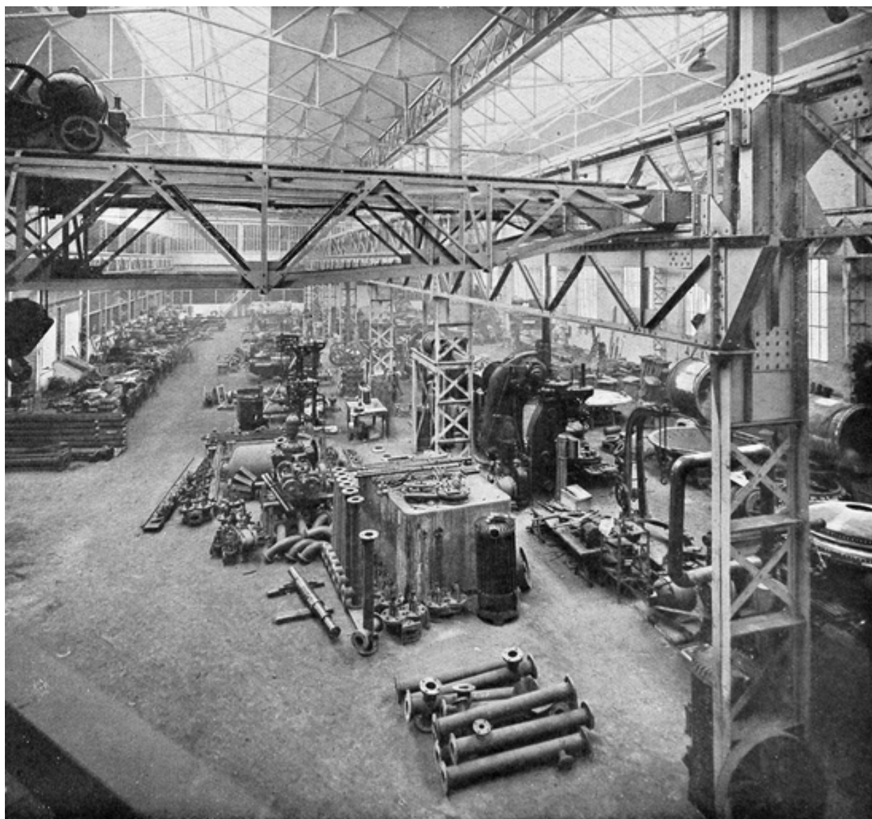
Un atelier de construction mécanique : matériel destiné à l'industrie sucrière, vers 1921 (Le Monde Illustré).
