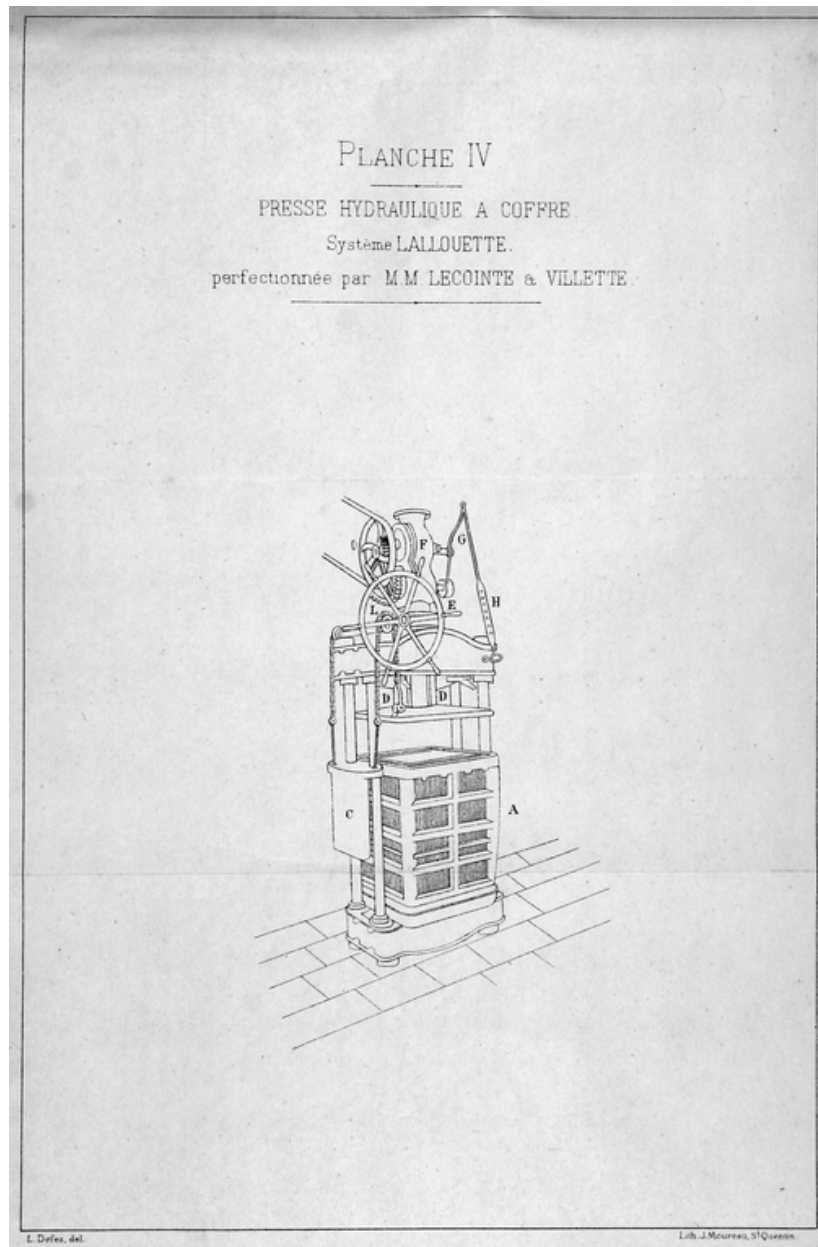
Presse hydraulique à coffre, Système Lallouette construite par Lecointe et Villette, 1878-1880 (Bulletin de la Société Industrielle de Saint-Quentin et de l'Aisne).
