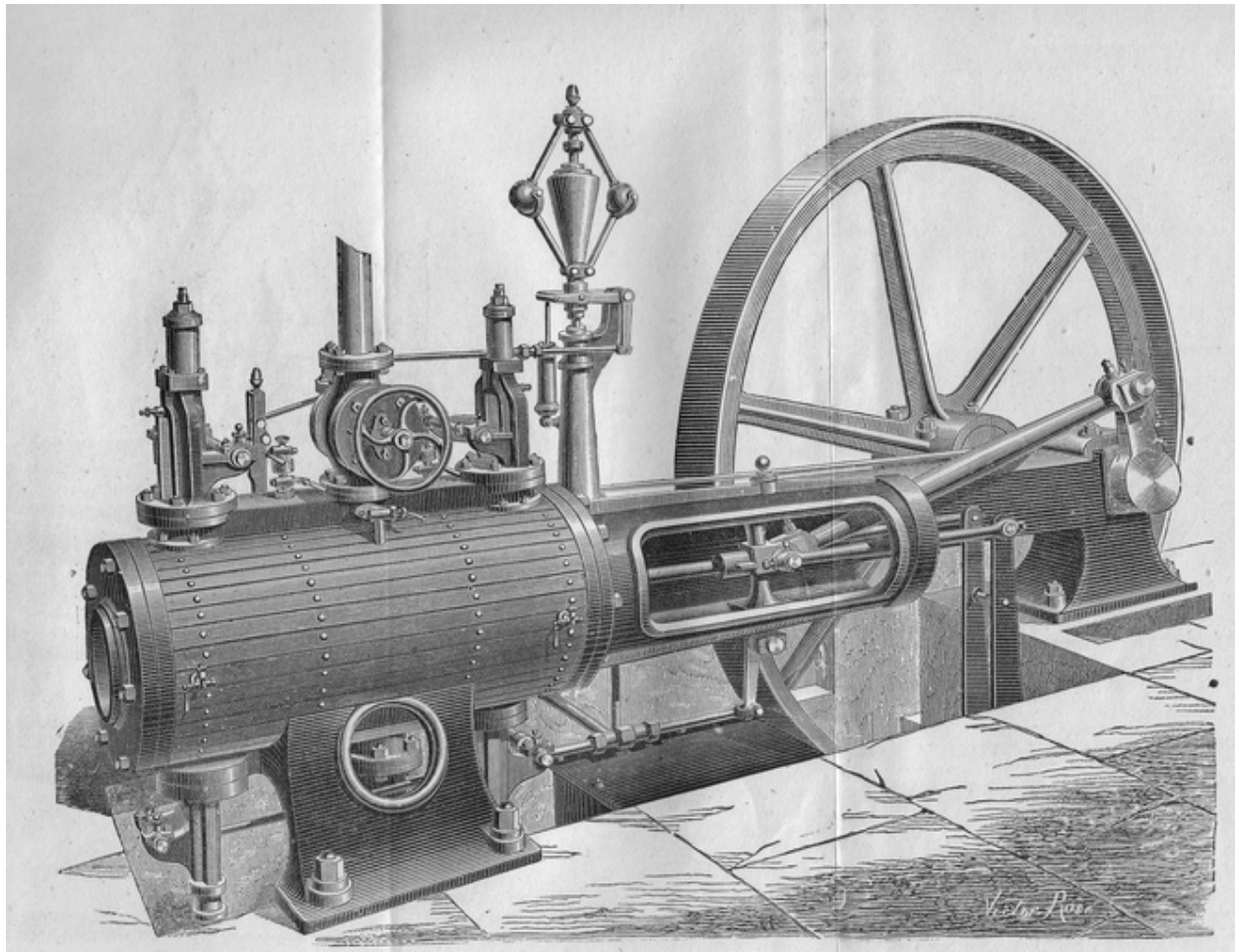
Machine à vapeur Zimmermann construite par Lecoigne & Villette, présentée à l'Exposition Universelle de 1878 (Bulletin de la Société Industrielle de Saint-Quentin et de l'Aisne).
