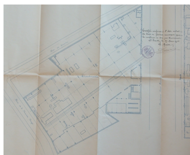
Plan des ateliers implantés à l'ouest du boulevard Henri-Martin (chaudronnerie), 1922 (AD Aisne). Phot. Pillet Frédéric IVR22_20050206033NUCAB
