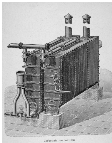
Appareil pour la carbonatation continue (industrie sucrière), vers 1900 (Le département de l'Aisne à l'Exposition Universelle de Paris en 1900).
