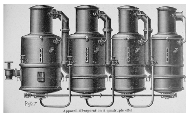
Appareil d'évaporation à quadruple effet, vers 1900 (Le département de l'Aisne à l'Exposition Universelle de Paris en 1900).
