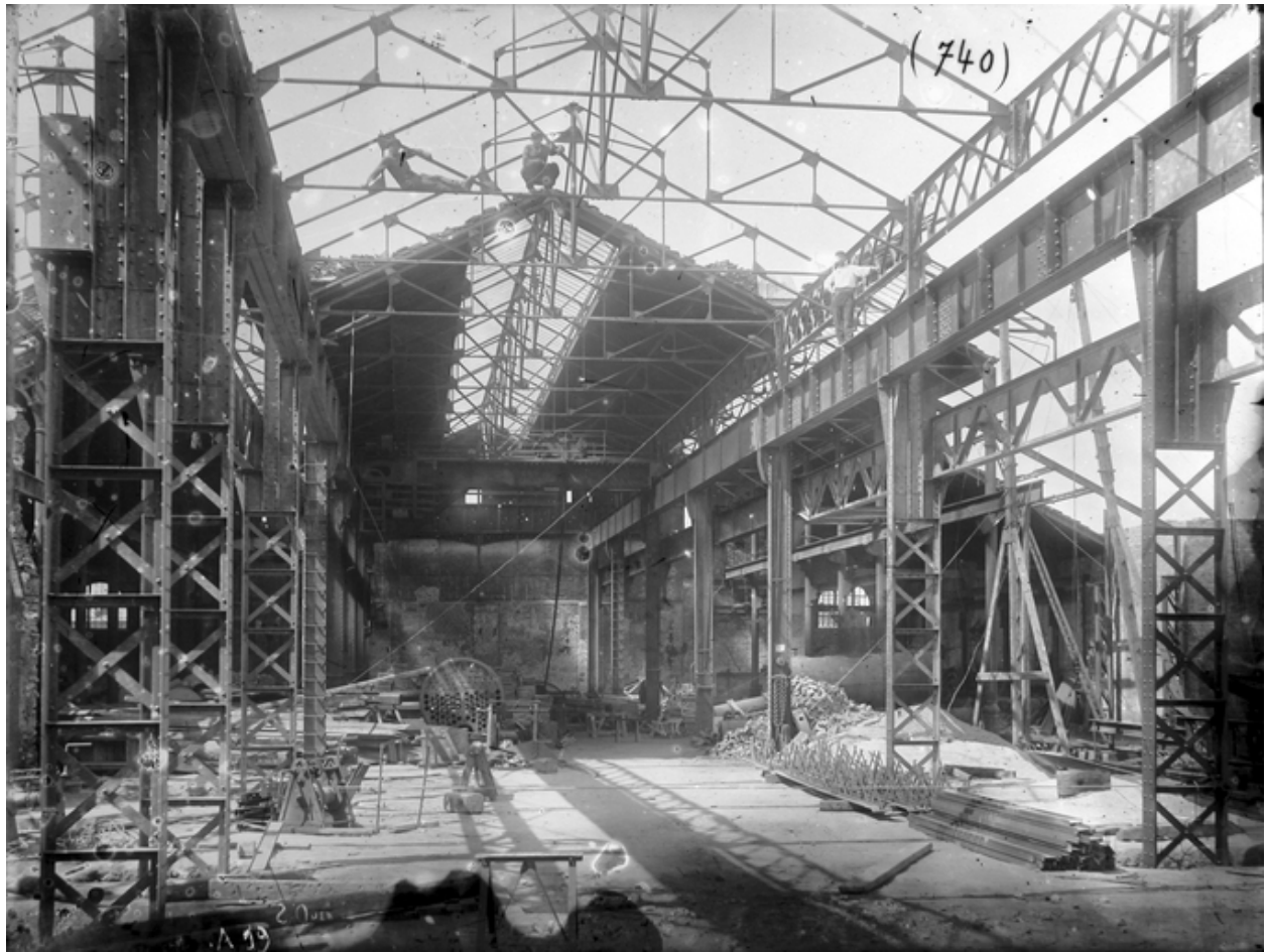
Les ateliers en cours de reconstruction, vers 1920-1921 (AD Aisne).
