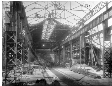
Les ateliers en cours de reconstruction, vers 1920-1921 (AD Aisne). Phot. Pillet Frédéric IVR22_20050206045NUCAB
