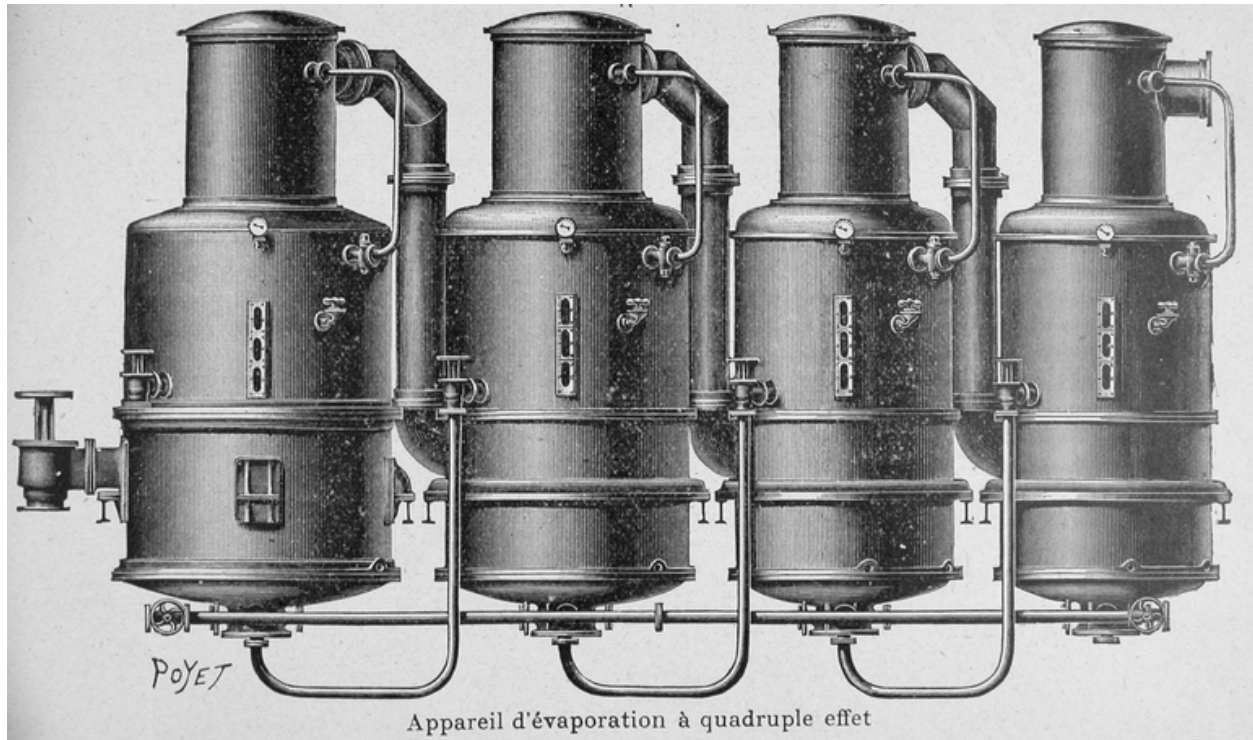
Appareil d'évaporation à quadruple effet, vers 1900 (Le département de l'Aisne à l'Exposition Universelle de Paris en 1900).
