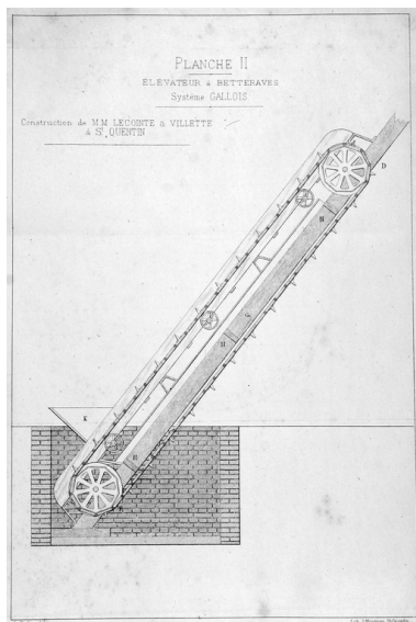
Elévateur à betteraves Système Gallois construit par Lecointe et Villette, 1878-1880 (Bulletin de la Société Industrielle de Saint-Quentin et de l'Aisne). Phot. Pillet Frédéric IVR22_20050206022NUCAB
