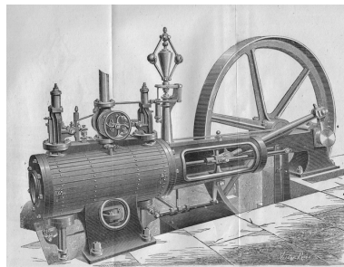
Machine à vapeur Zimmermann construite par Lecointe & Villette, présentée à l'Exposition Universelle de 1878 (Bulletin de la Société Industrielle de Saint-Quentin et de l'Aisne). Phot. Pillet Frédéric IVR22_20050206029NUCAB
