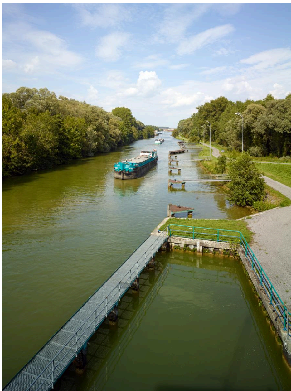
Vue en aval de l'écluse. Estacade de guidage, passerelle métallique, bassin de tranquillisation. Appontements type "Duc d'Albe".
