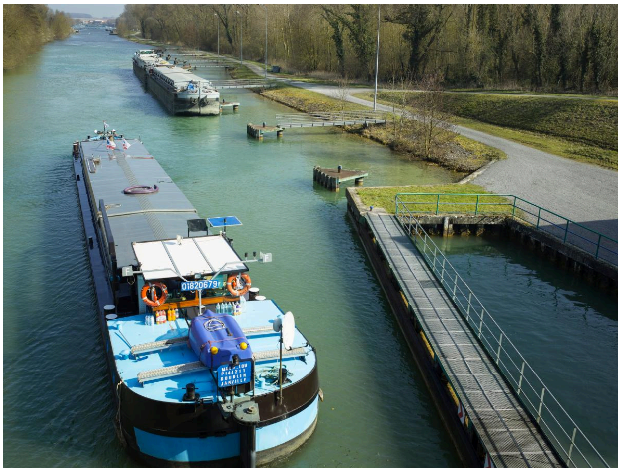
Estacade de guidage et appontements à l'aval. La péniche Freycinet "Marie-Lou" sortant de l'écluse et se dirigeant vers la jonction Sensée-canal de Dunkerque-Valenciennes. En arrière-plan, le convoi poussé "Kenza".
