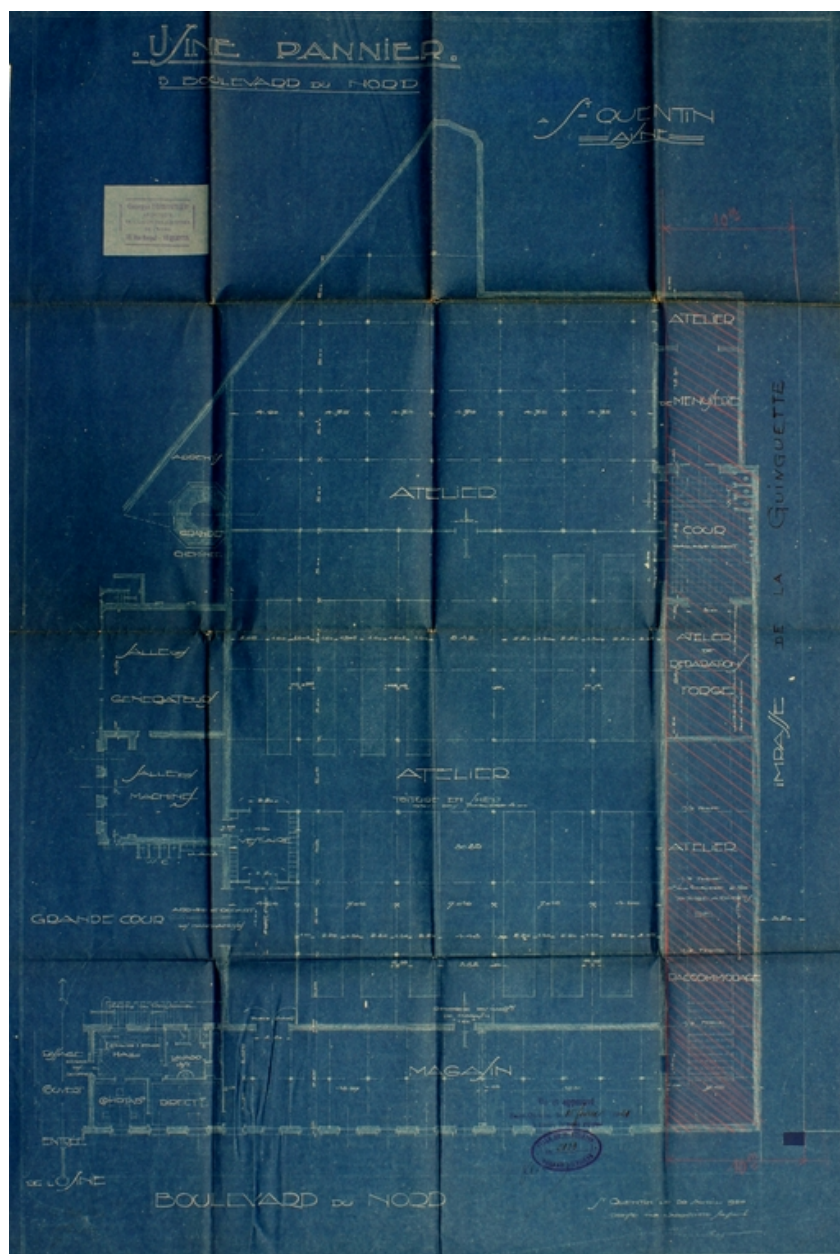
Usine Pannier. Plan de l'usine, par Dumortier, 1920 (AC Saint-Quentin).
