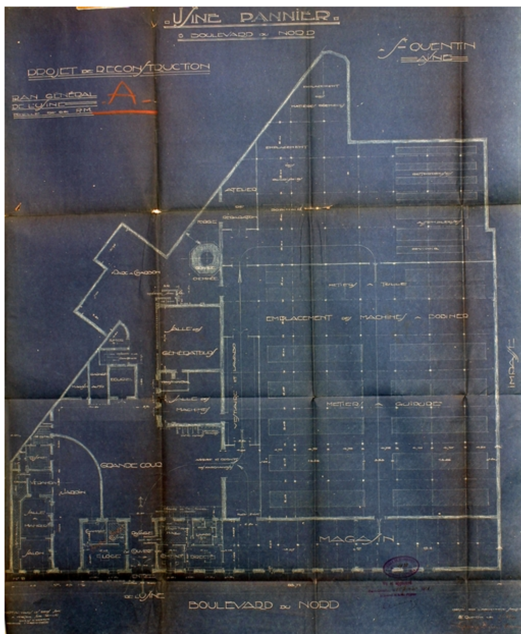
Usine Pannier. Projet de reconstruction A, par Dumortier, 1920 (AC Saint-Quentin).
