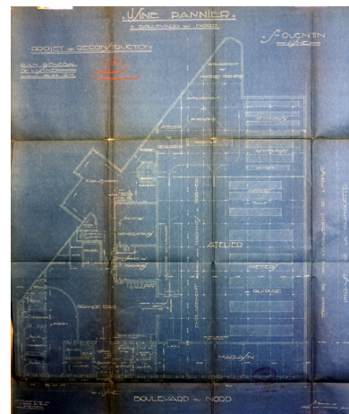
Usine Pannier. Projet de reconstruction B, par Dumortier, 1920 (AC Saint-Quentin). Phot. Pillet Frédéric IVR22_20040200651NUCAB
