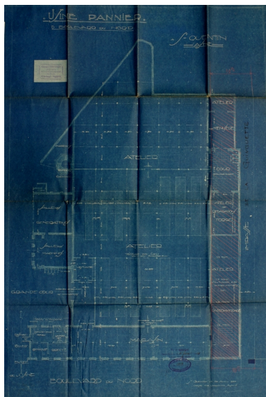
Usine Pannier. Plan de l'usine, par Dumortier, 1920 (AC Saint-Quentin). Phot. Pillet Frédéric IVR22_20040200649NUCAB
