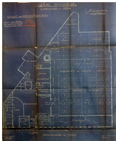
Usine Pannier. Projet de reconstruction A, par Dumortier, 1920 (AC Saint-Quentin). Phot. Pillet Frédéric IVR22_20040200650NUCAB
