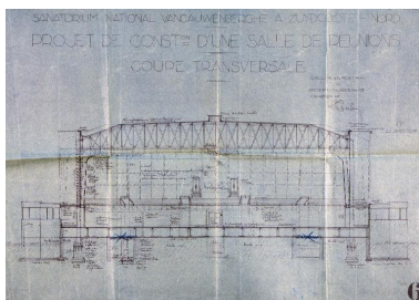
Salle des fêtes, coupe transversale, non datée, vers 1932 ou 1933 (IFA). Autr. Roger Poulain, Repro. Pierre Thibaut IVR31_20125901507NUCA
