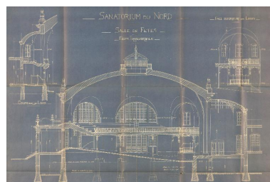
Salle des fêtes, coupe transversale, datée du 20 mars 1906 (IFA). Repro. Pierre Thibaut IVR31_20125901509NUCA
