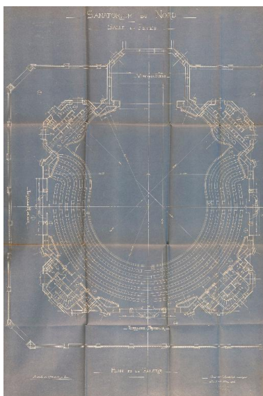
Salle des fêtes, plan de distribution au niveau des tribunes, datée du 20 mars 1906 (IFA). Repro. Pierre Thibaut IVR31_20125901511NUCA
