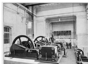
Bâtiment des machines, salle des générateurs, vue générale, photographie ancienne (archives de l'établissement). Repro. Philippe Dapvril IVR31_20035900219XB
