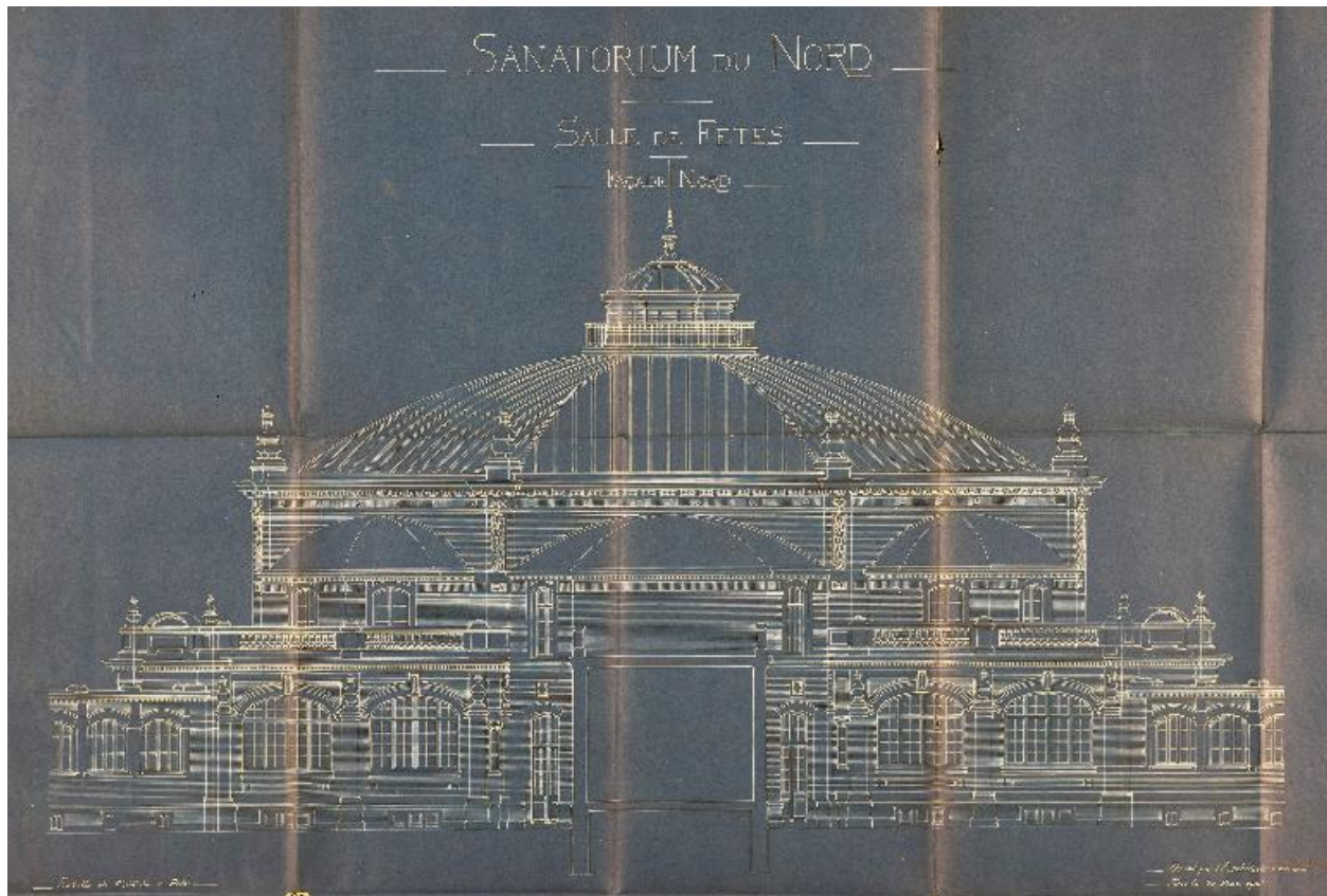
Salle des fêtes, élévation septentrionale, datée du 20 mars 1906 (IFA).
