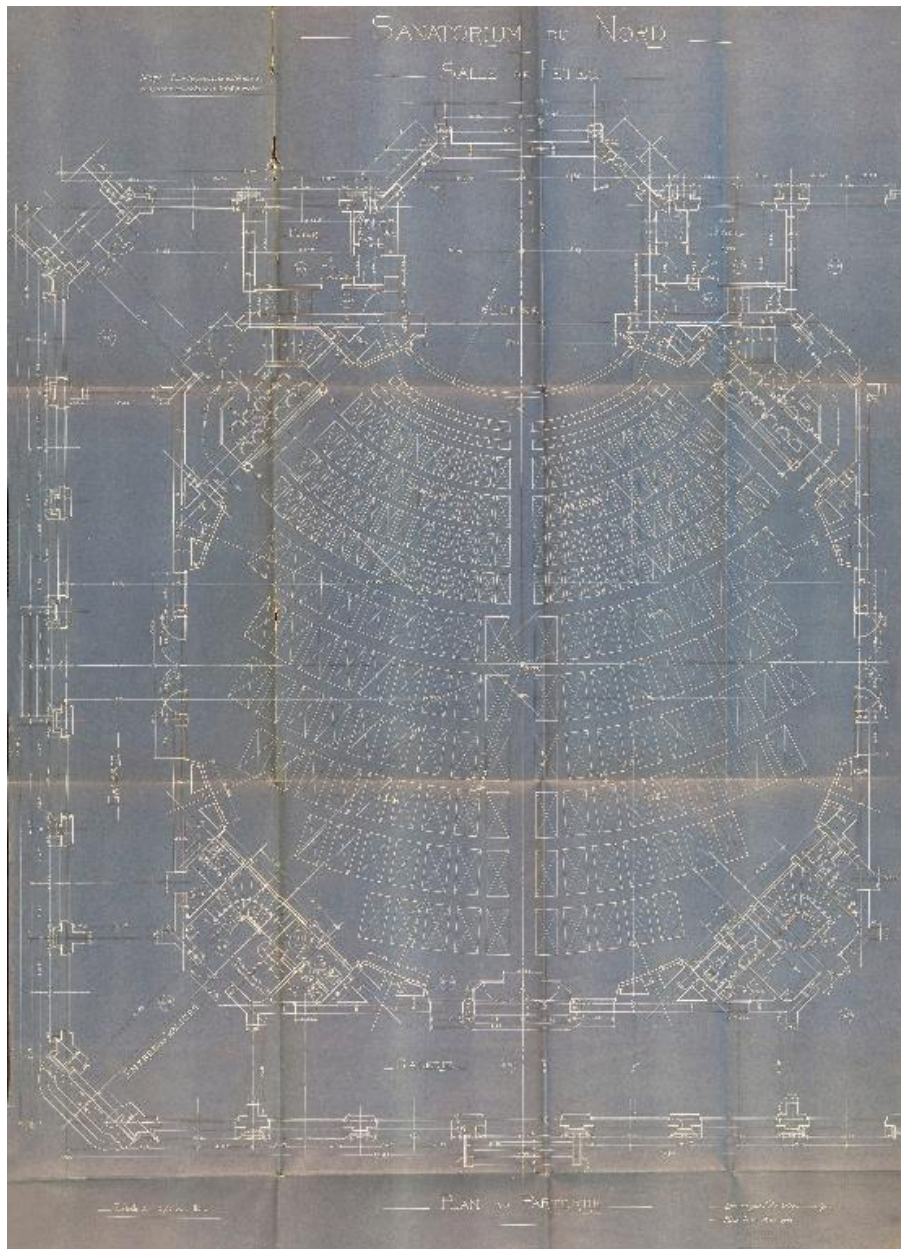
Salle des fêtes, plan de distribution au niveau du parterre, datée du 20 mars 1906 (IFA).
