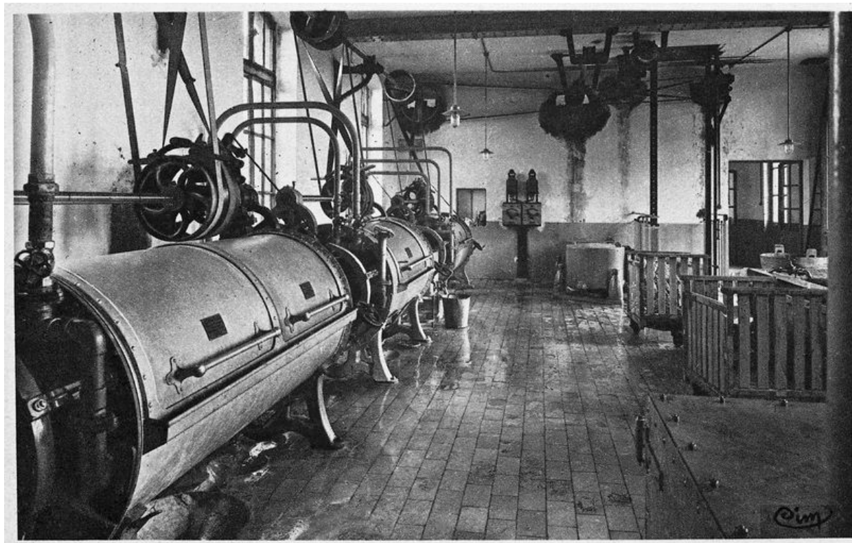
Bâtiment des machines, blanchisserie, vue en enfilade des lessiveuses-autoclaves, photographie ancienne (archives de l'établissement).
