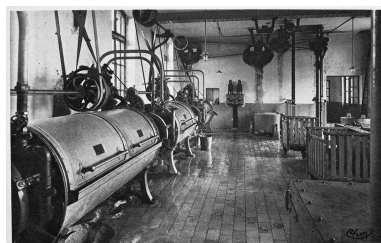
Bâtiment des machines, blanchisserie, vue en enfilade des lessiveuses-autoclaves, photographie ancienne (archives de l'établissement). Repro. Philippe Dapvril IVR31_20035900218XB
