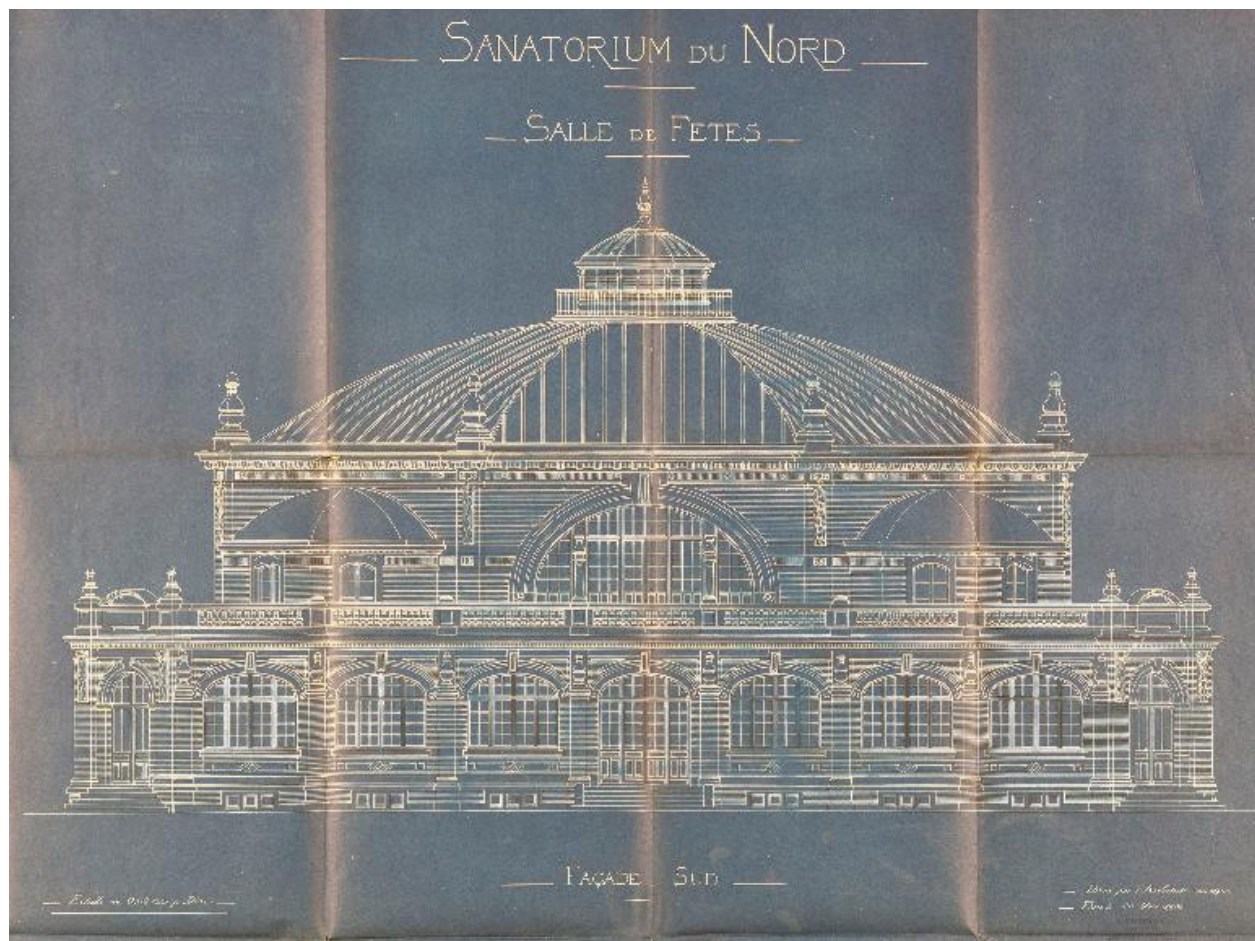
Salle des fêtes, élévation méridionale, datée du 20 mars 1906 (IFA).
