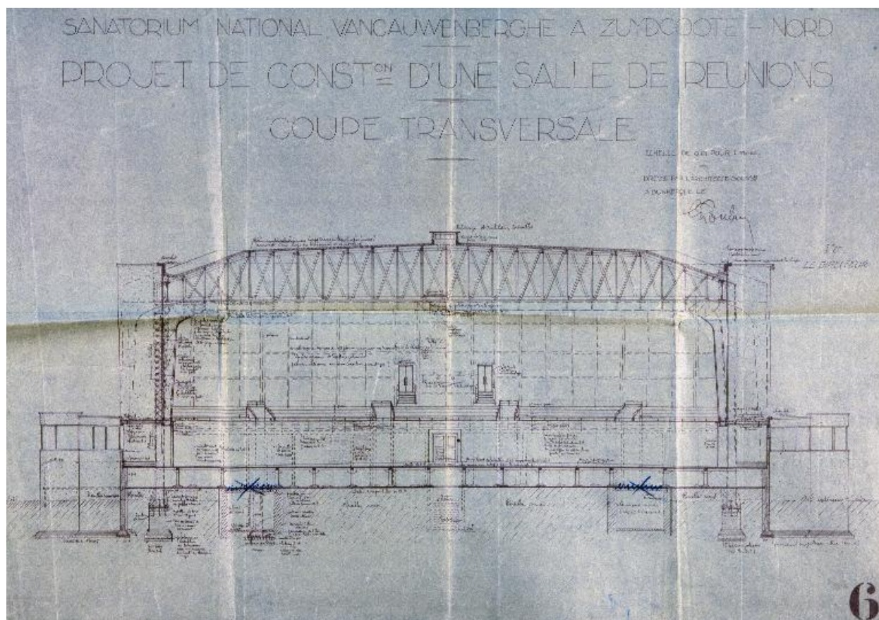
Salle des fêtes, coupe transversale, non datée, vers 1932 ou 1933 (IFA).
