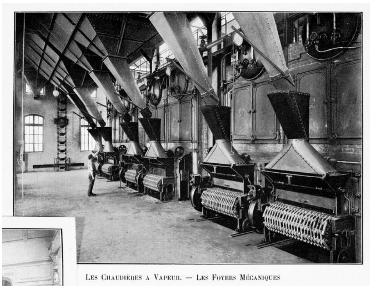
Bâtiment des machines, salle des chaudières, vue en enfilade des chaudières à vapeur, photographie ancienne (archives de l'établissement).
