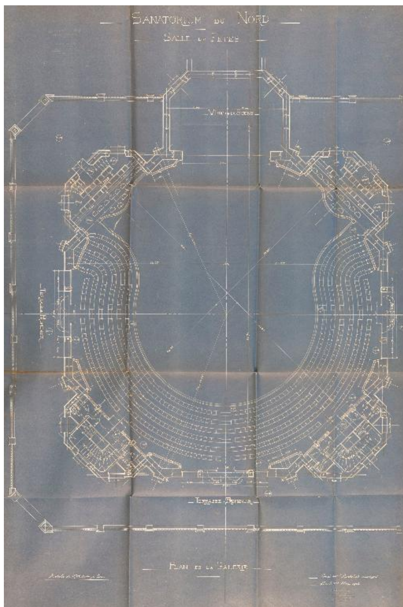
Salle des fêtes, plan de distribution au niveau des tribunes, daté du 20 mars 1906 (IFA).
