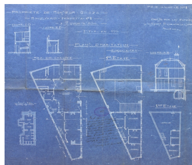
Plan du logement patronal, par Brassart-Mariage, 1914 (AC Saint-Quentin). Phot. Pillet Frédéric IVR22_20050206172NUCAB
