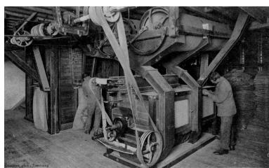
L'usine de semence Léon Legland, carte postale n°6 : une batterie de trieurs pour blés, avoine, carte postale sans date (Archives privées). Phot. Pierre Thibaut IVR31_20085900476NUC
