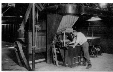
L'usine de semence Léon Legland, carte postale n°7 : batteuse et appareil de réglage de densité du grain, carte postale sans date (Archives privées). Phot. Pierre Thibaut IVR31_20085900477NUC
