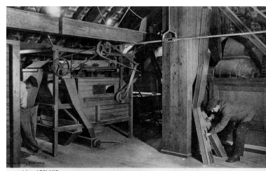
L'usine de semence Léon Legland, carte postale n°5 : tarrare et aspirateur pour blés et avoine, carte postale sans date (Archives privées).
