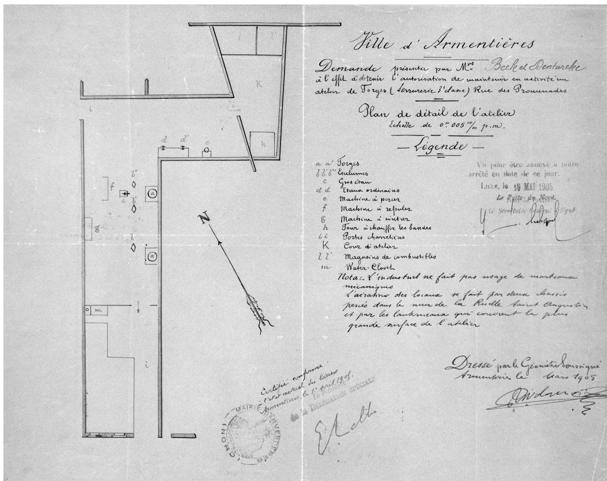
Beck et Denturcke. Demande de maintien en activité d'usine de serrurerie. Plan masse, 1905 (AD Nord ; M 4175333).
