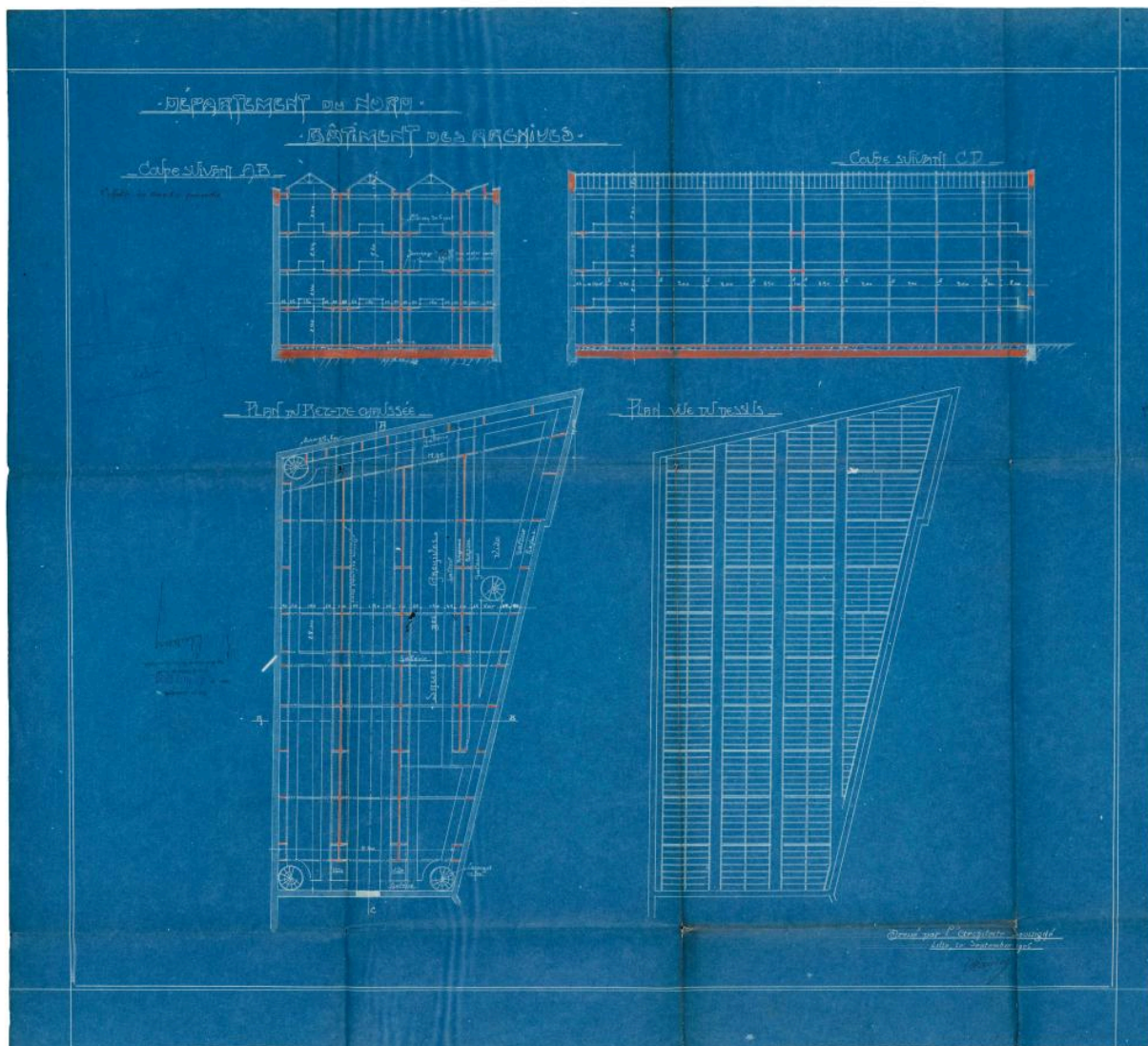
Plans et coupes du bâtiment du dépôt (projet) par Léonce Hainez, septembre 1906 (AD Nord ; 4 N 232).
