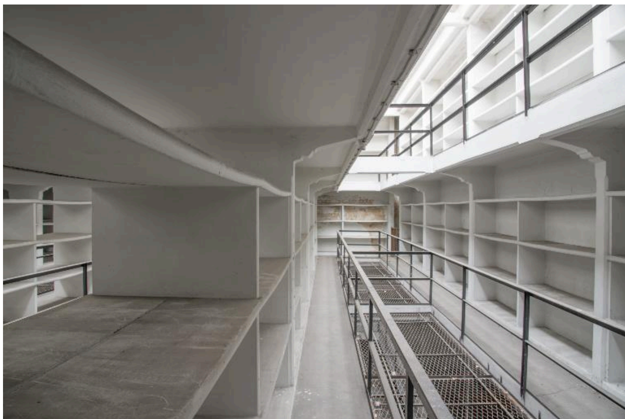
Bâtiment du dépôt, deuxième étage : vue des rayonnages entre les vaisseaux 1 et 2. À noter : l'absence de cloison verticale qui garantit une bonne circulation de l'air derrière les liasses.
