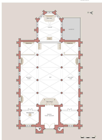
Plan de l'église Saint-Denis de Noordpeene. Dess. Eddy Stein IVR32_20265900062NUDA
