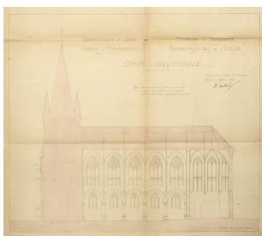
Reconstruction de l'église de Noordpeene. Coupe longitudinale. Dressée par l'architecte Maillard le 10 juin 1894 (AD Nord : 2 O 437/18). Repro. Delphine Volto Jourdan, Phot. Jean-Baptiste Maillard IVR32_20255900554NUCA
