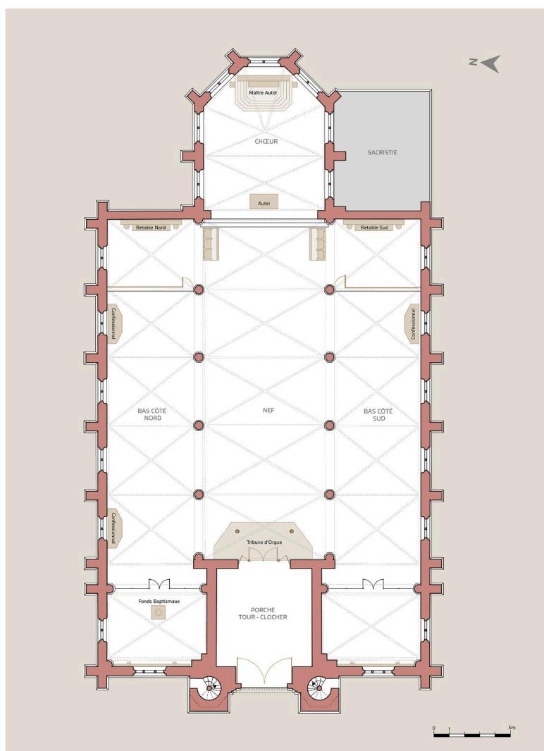
Plan de l'église Saint-Denis de Noordpeene.
