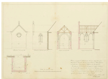
Plan, coupes et élévations d'une chapelle que monsieur Ernest Duvet(...) à l'intention d'annexer à l'église de Noordpeene. Dressés par l'architecte Outters le 4 février 1880 (AD Nord : 2 O 437/17). Repro. Delphine Volto Jourdan, Phot. Auguste Outters IVR32_20255900553NUCA
