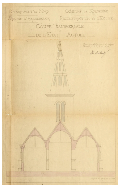
Ancienne église de Noordpeene - coupe transversale de l'église actuelle. Dressée par l'architecte Maillard le 10 juin 1894 (AD Nord : 2 O 437/18).
