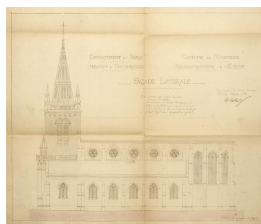
Reconstruction de l'église de Noordpeene. Façade latérale. Plan dressé par l'architecte Maillard le 10 juin 1894 (AD Nord : 2 O 437/18). Repro. Delphine Volto Jourdan, Phot. Jean-Baptiste Maillard IVR32_20255900555NUCA
