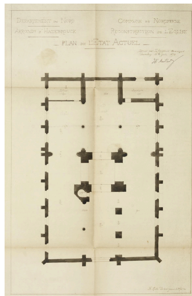
Ancienne église de Noordpeene - plan de l'église actuelle. Dressé par l'architecte Maillard le 10 juin 1894 (AD Nord : 2 O 437/18). Repro. Delphine Volto Jourdan, Phot. Jean-Baptiste Maillard IVR32_20255900558NUCA
