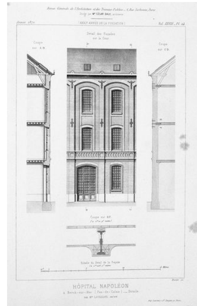
Détail de l'élévation de deux travées et coupe transversale partielle d'un des bâtiments d'hébergement des enfants valétudinaires. Rev. gén. de l'arch., t. XXVIII, pl. 24. Phot. Pierre Thibaut IVR31_20086200261X
