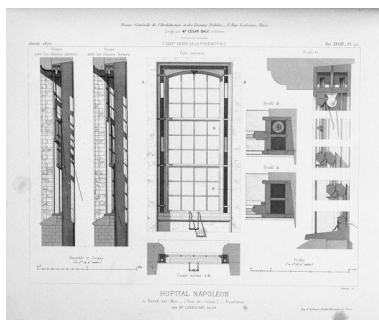
Dessin de l'huissier d'une fenêtre en coupes et en élévation avec des détails de l'assemblage des bois. Rev. gén. de l'arch., t. XXVIII, pl. 25. Phot. Pierre Thibaut IVR31_20086200260X
