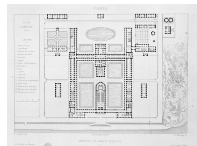
Plan de distribution générale légendé du rez-de-chaussée. NARJOUX, F. Paris, monuments élevés par la ville, tome IV, planche non numérotée. Phot. Pierre Thibaut IVR31_20086200258X
