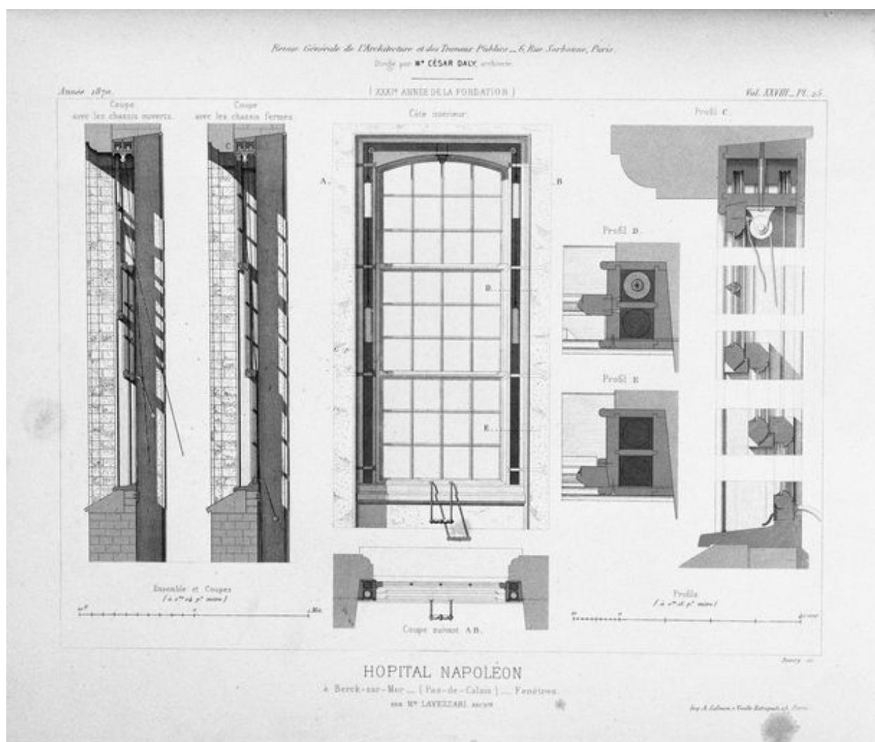
Dessin de l' huisserie d'une fenêtre en coupes et en élévation avec des détails de l'assemblage des bois. Rev. gén. de l'arch., t. XXVIII, pl. 25.
