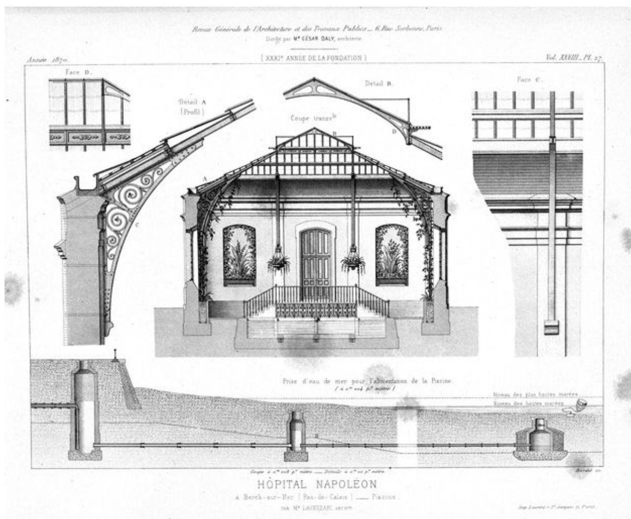
Piscine d'eau de mer couverte, coupe transversale, détails de la structure métallique du couvrement et coupe du système de prise d'eau de mer pour l'alimentation du bassin. Rev. gén. de l'arch., t. XXVIII, pl. 27.
