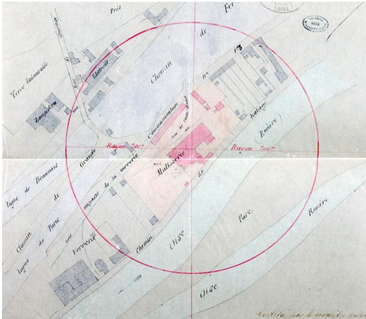
Localisation de la verrerie établie par Garchey en 1898, plan dressé par Depas géomètre (AD Oise ; 5Mp2456/2).
