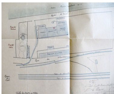
Plan de la malterie, par Péroche, en 1887 (AD Oise ; 5Mp2455/1).
