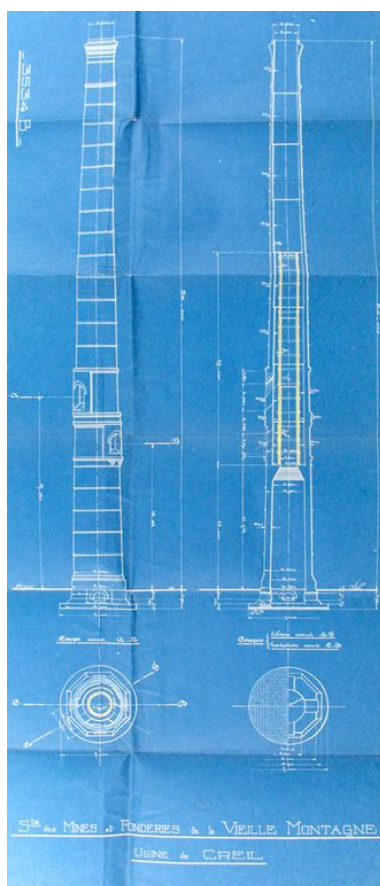
Plan des cheminées construites en 1923 (AD Oise ; 5Mp2457). Phot. Clarisse Lorieux IVR22_20076005145NUCAB
