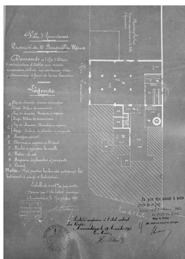
Bouquillon-Wgeux. Installation d'une scierie mécanique. Plan masse, 1891 (AD Nord ; M 417 537). Repro. Philippe Dapvril IVR31_19875902317X
