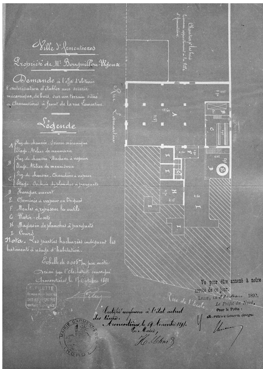
Bouquillon-Wgeux. Installation d'une scierie mécanique. Plan masse, 1891 (AD Nord ; M 417 537).
