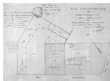
Bouquillon-Wgeux. Dépôt de matières bitumeuses solides. Plan masse, 1905 (AD Nord, M 417536). Repro. Philippe Dapvril IVR31_19875902375X
