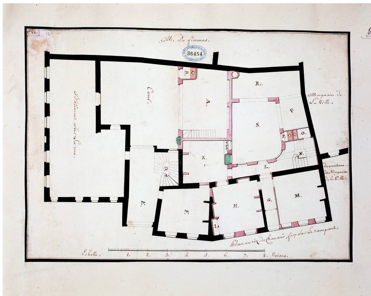
Plan de masse. B.M. Boulogne-sur-Mer, 13e portefeuille, fol. 22.
