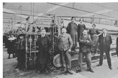
Une partie du personnel de l'usine posant devant une machine à broder à fil continu installée à la reconstruction, vers 1920-1922 (Le Monde Illustré). Phot. Pillet Frédéric IVR22_20040200610NUCAB
