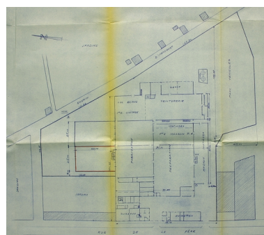
Plan masse de l'usine, 1966 (AC Saint-Quentin).
