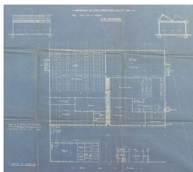
Plan du tissage de Saint-Quentin en 1920, par Malgras-Delmas (AD Aisne).
