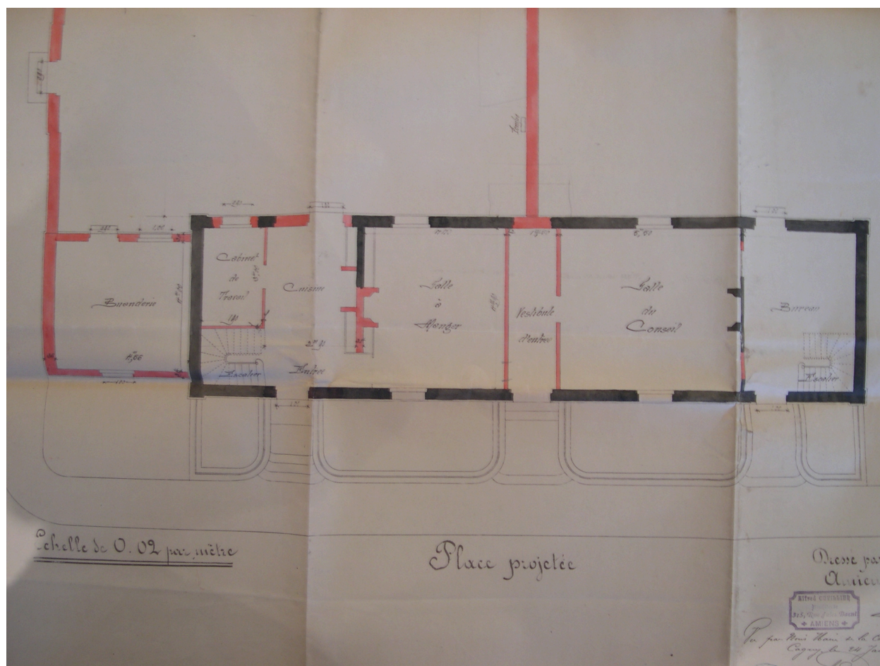
Cagny. Construction d'une école de garçons. Plan du rez-de-chaussée, dessin, Alfred Cuvillier architecte, 1902 (AD Somme ; 99 O 985).
