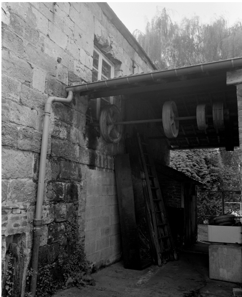
Système de poulies par courroies installé entre la salle des machines et l'atelier de fabrication en pierre de taille.
